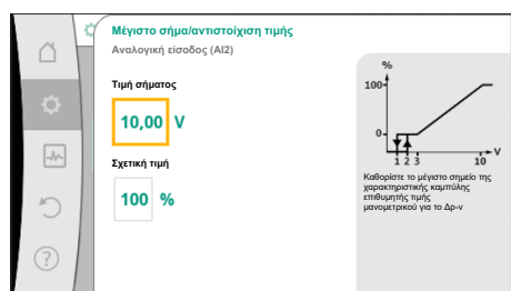
Fig. 83: Μέγιστο σήμα/αντιστοίχιση τιμής
