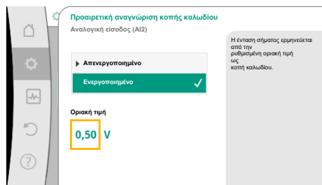
Fig. 79: Οριακή τιμή κοπής καλωδίου
