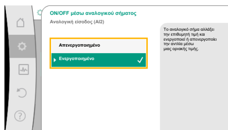
Fig. 80: ON/OFF μέσω αναλογικού σήματος
