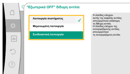
Fig. 66: Επιλεγόμενες λειτουργίες για EXT. OFF σε διδυμες αντλίες
