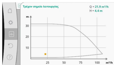
Fig. 96: Τρέχον σημείο λειτουργίας
