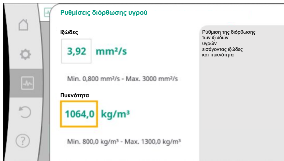
Fig. 98: Ρύθμιση ιξώδους και πυκνότητας
