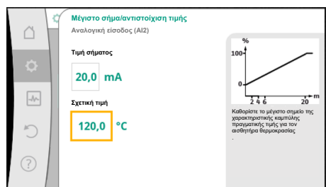
Fig. 88: Μέγιστο σήμα/αντιστοίχιση τιμής δότη πραγματικής τιμής
