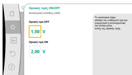
Fig. 81: Οριακές τιμές για τον έλεγχο ON/OFF μέσω αναλογικών σημάτων
