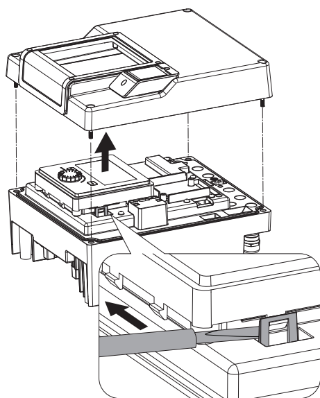
Fig. 113: Αφαιρέστε το κάλυμμα μονάδας. Χαλαρώστε τη μονάδα οθόνης και χειρισμού από την ασφάλιση
