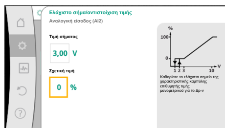
Fig. 82: Ελάχιστο σήμα/αντιστοίχιση τιμής
