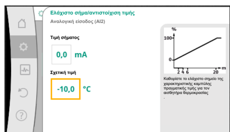
Fig. 87: Ελάχιστο σήμα/αντιστοίχιση τιμής δότη πραγματικής τιμής
