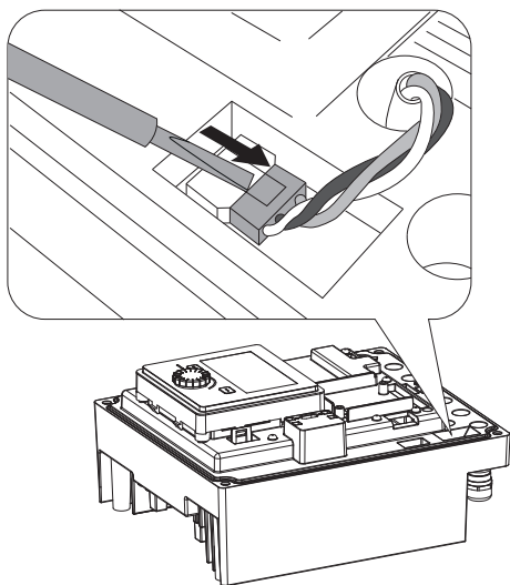
Fig. 110: Ξεσφίξτε το καλώδιο σύνδεσης του ανεμιστήρα στοιχείου
