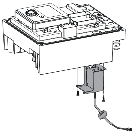
Fig. 112: Αφαιρέστε τον ανεμιστήρα στοιχείου μαζί με το καλώδιο και την ελαστική στεγανοποίηση
