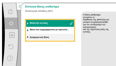
Fig. 70: Επιλογή θέσης αισθητήρα
