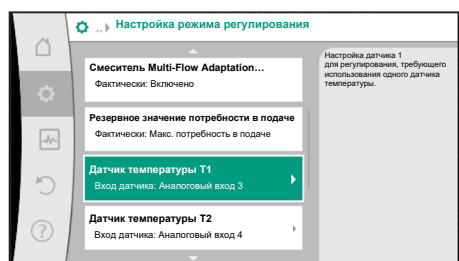
Fig. 62: Смеситель Multi-Flow Adaptation: датчик температуры
