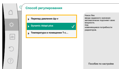
Fig. 43: Пример способа регулирования Dynamic Adapt plus
