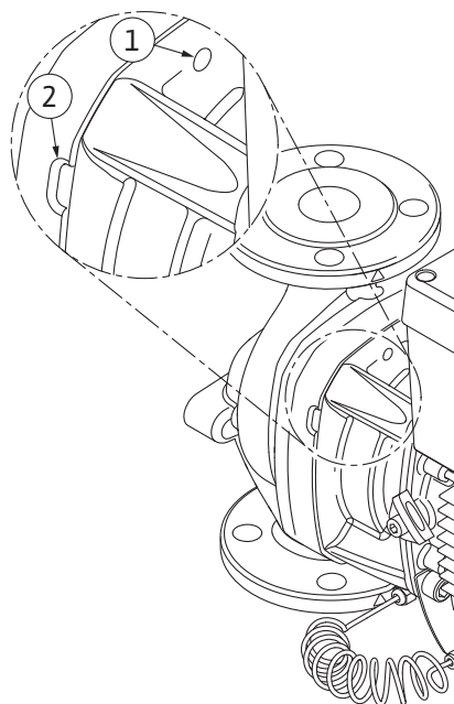
Fig. 105: Резьбовые отверстия и шлицы для отжатия съемного блока от корпуса насоса
