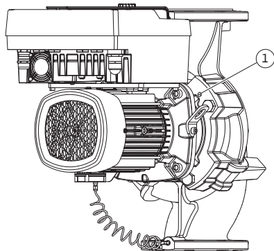
Fig. 104: Отжатие съемного блока через резьбовые отверстия
