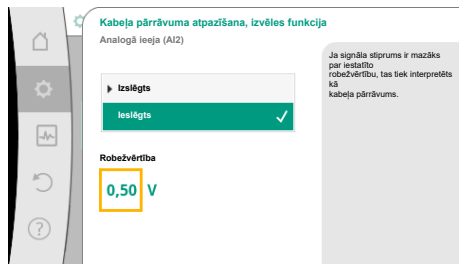
Fig. 79: Robežvērtība, kabeļa pārvērtums
