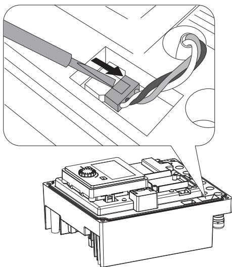
Fig. 110: Moduļa ventilatora pieslēguma kabeļa atvienošana
