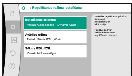
Fig. 44: Iestatīšanas asistents
