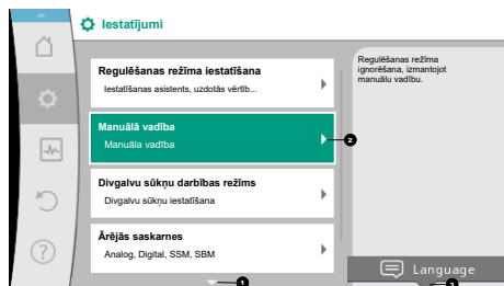
Fig. 35: Iestatījumu izvēlne
