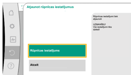
Fig. 101: Rūpnīcas iestatījums
