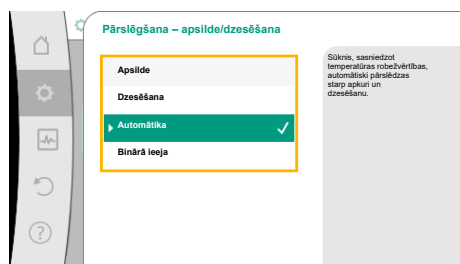
Fig. 51: Pārslēgšana – apsilde/dzesēšana_Automātika
