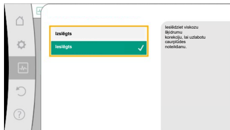
Fig. 97: Šķidrumu korekcija
