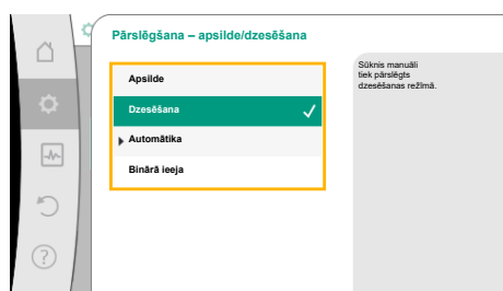
Fig. 50: Pārslēgšana – apsilde/dzesēšana_Dzesēšana
