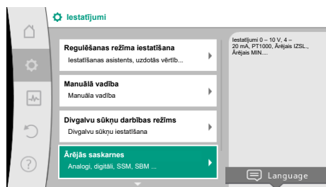
Fig. 67: Ārējās saskarnes
