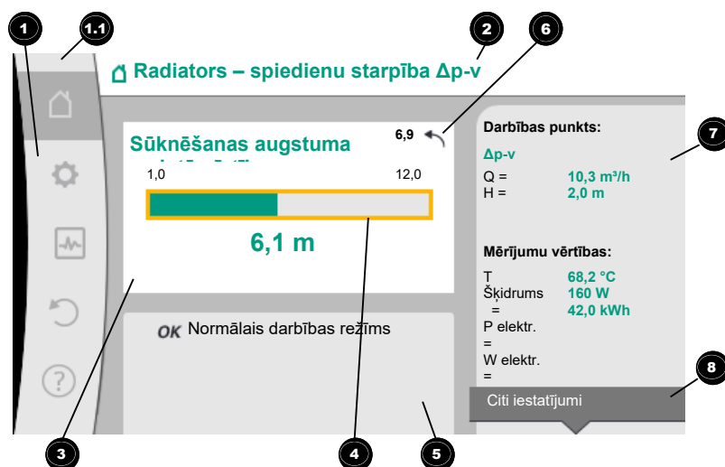
Fig. 34: Sākuma ekrāns
