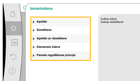
Fig. 40: Pielietojuma izvēle
