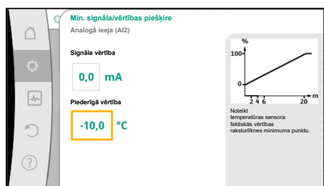
Fig. 87: Min. signāla/vērtības piešķiršana, faktiskās vērtības devējs
