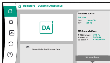
Fig. 33: Galvenā izvēlne
