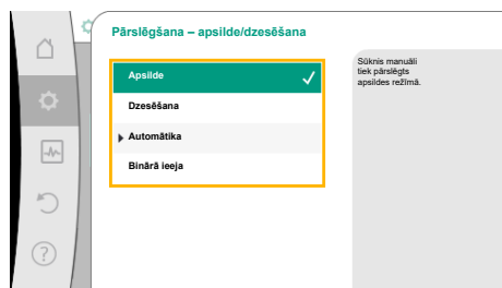
Fig. 49: Pārslēgšana – apsilde/dzesēšana_Apsilde
