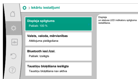
Fig. 91: Iekārtu iestatījumi
