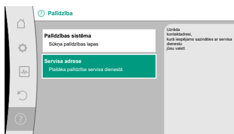
Fig. 103: Servisa adrese
