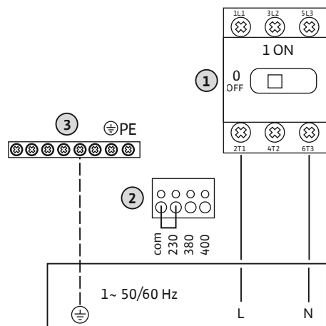
Fig. 4: Netaansluiting Control EC-rF
