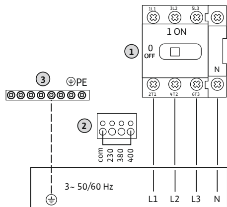
Fig. 5: Netaansluiting Control EC-rh
