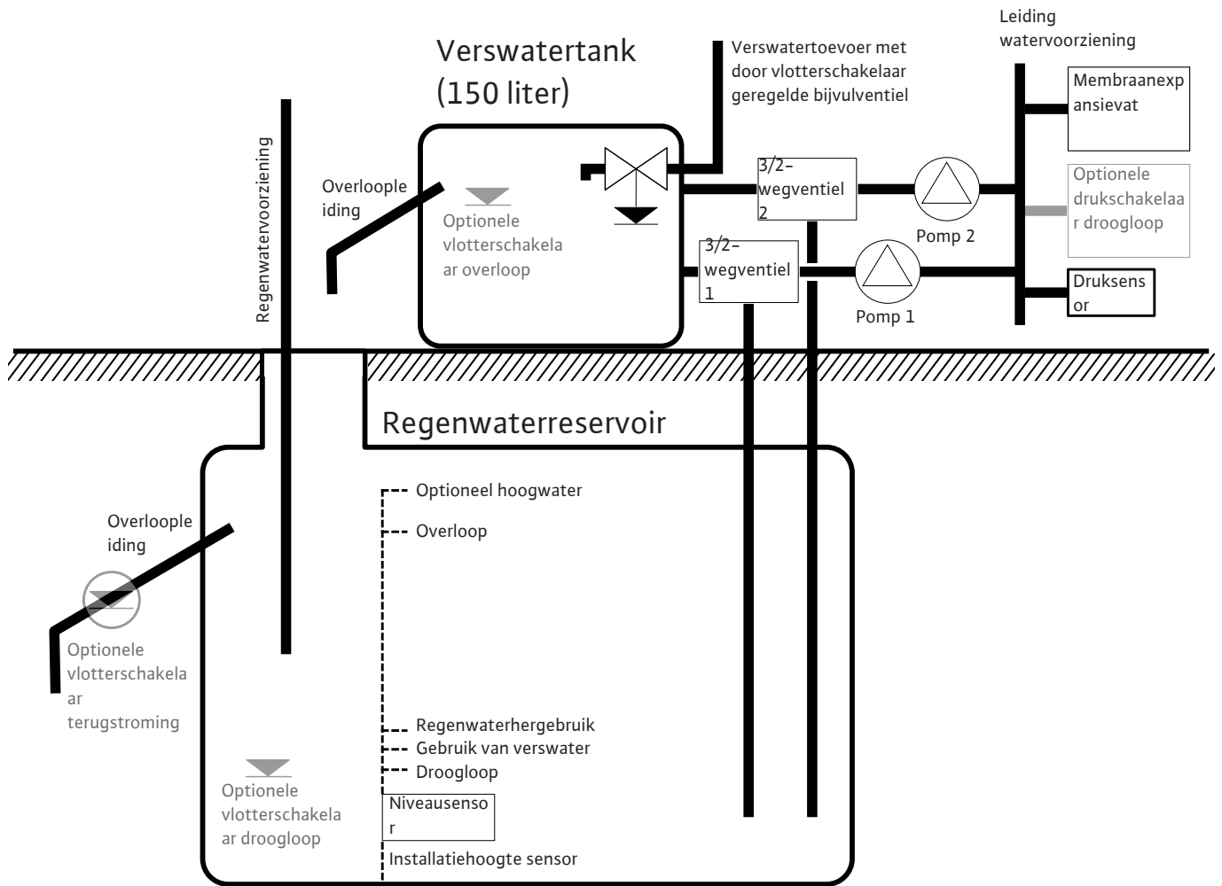
Fig. 22: Werkingsprincipe van de AF150 schematisch weergegeven
