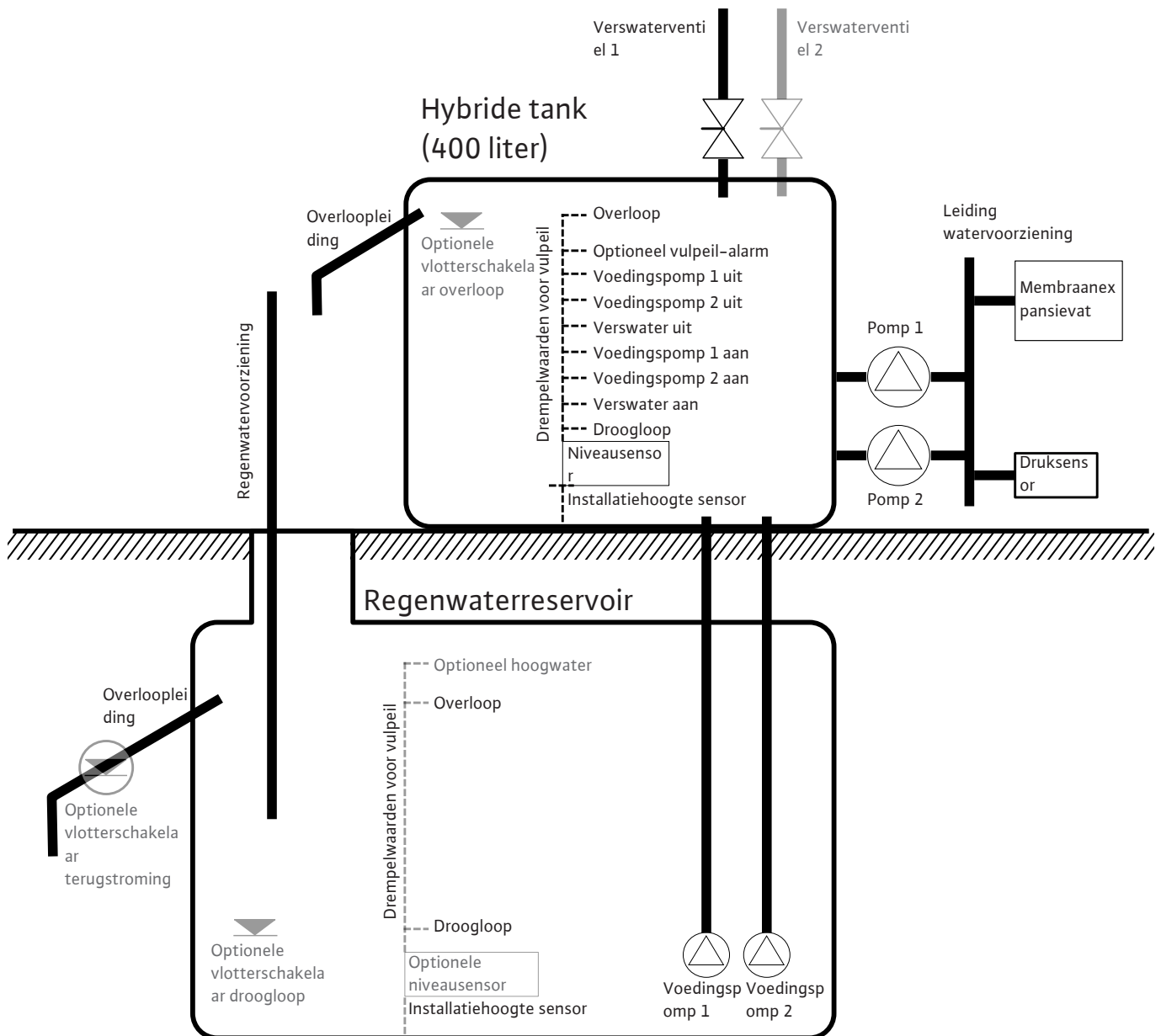
Fig. 23: AF400 werkingsprincipe met niveausensor in de hybride tank en in het regenwaterreservoir
