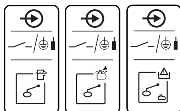
Fig. 12: Symbool-overzicht van de aansluitingen
