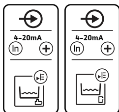
Fig. 11: Symbool-overzicht van de aansluitingen
