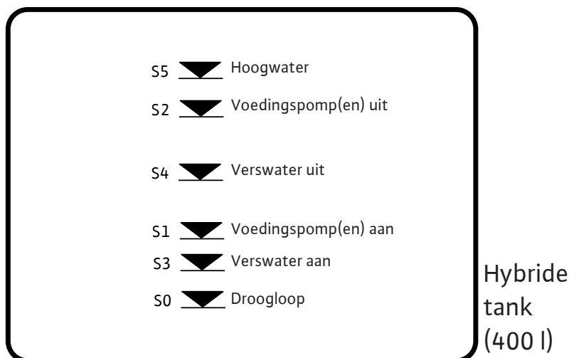
Fig. 26: Bedrijf met niveausensor
