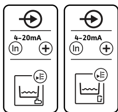
Fig. 11: Σύμβολο επισκόπησης σύνδεσης
