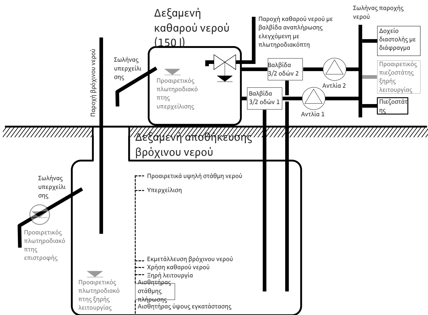
Fig. 22: Σχηματική απεικόνιση της αρχής λειτουργίας του συστήματος AF150
