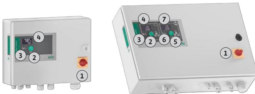
Fig. 1: Πρόσοψη ηλεκτρικού πίνακα, αριστερά ηλεκτρικός πίνακας EC-rF, δεξιά ηλεκτρικός πίνακας EC-rh + EC-Booster
