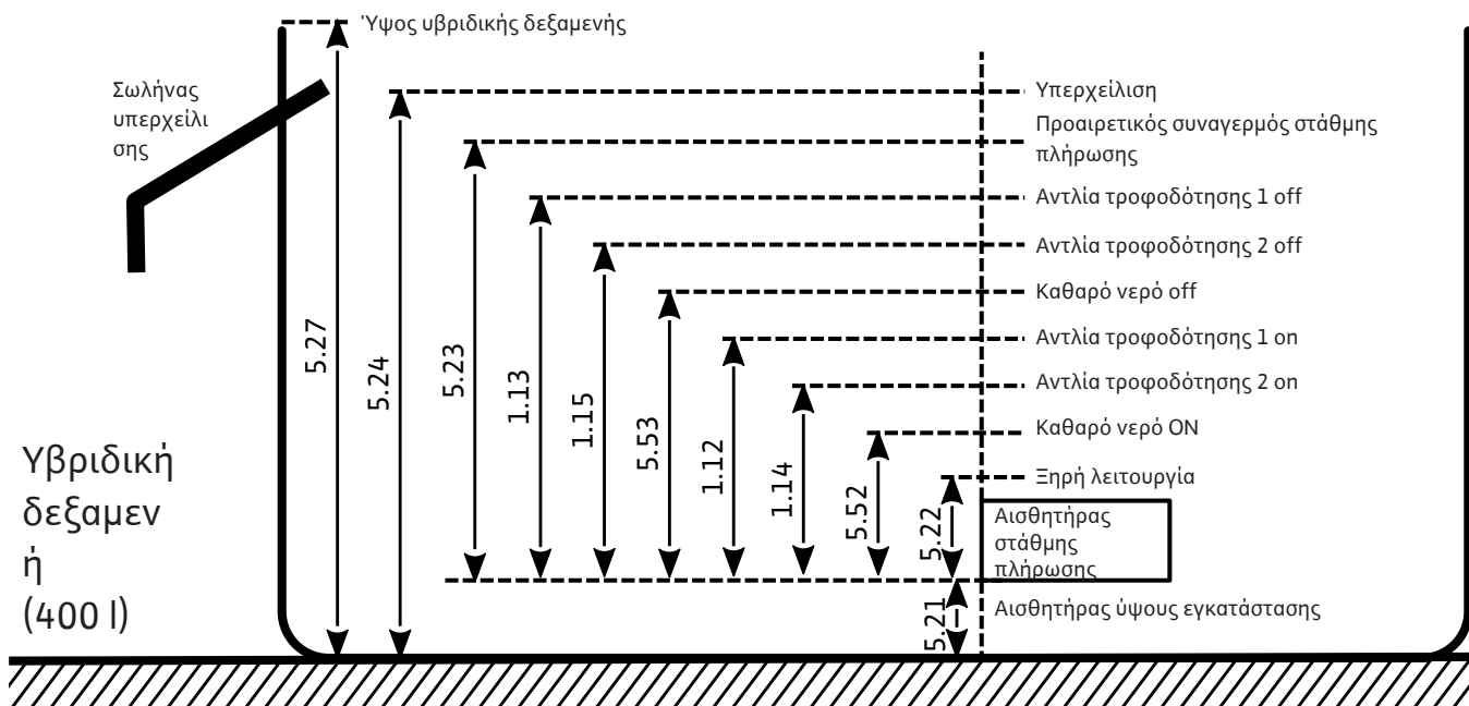
Fig. 25: Παράμετροι ρύθμισης υβριδικής δεξαμενής
