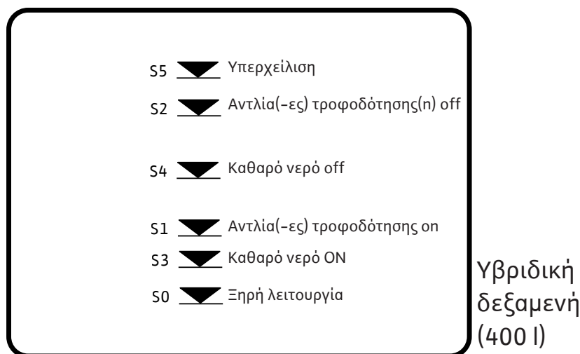
Fig. 26: Λειτουργία με αισθητήρα στάθμης
