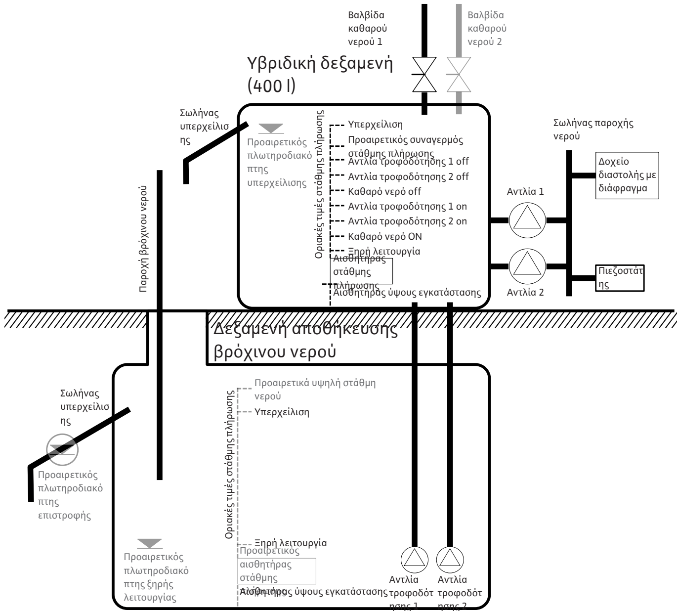
Fig. 23: AF400 Αρχή λειτουργίας με αισθητήρα στάθμης πλήρωσης στην υβριδική δεξαμενή και στη δεξαμενή αποθήκευσης βρόχινου νερού
