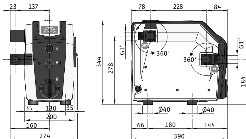
Fig. 3: Dimensões
