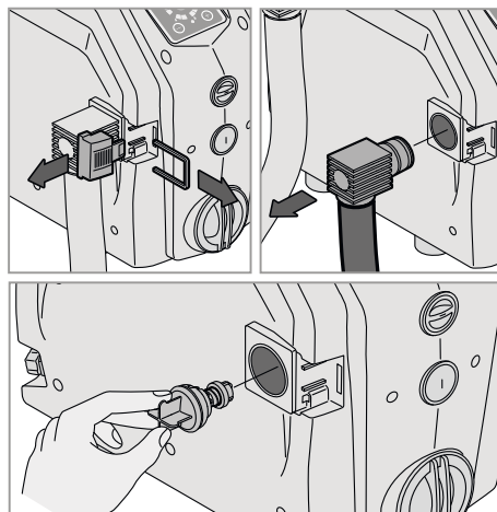
Fig. 16: Ligação de sucção do dispositivo de afluxo
