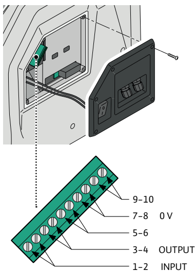
Fig. 6: Ligações do cartão de extensão
