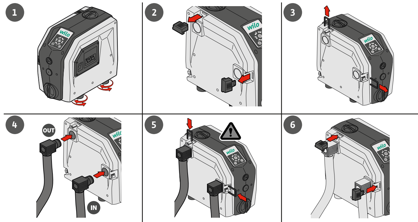
Fig. 5: Ligação hidráulica
