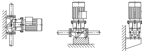
Fig. 4: Vista IPL - Instalação sobre fundações (≤ 7,5 kW)
