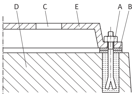
Fig. 9: Παράδειγμα για κοχλίωση θεμελίωσης
