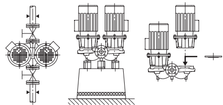
Fig. 5: Όψη DPL
