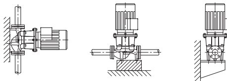
Fig. 4: Όψη IPL - Θεμελίωση ( \leq 7,5 kW)
