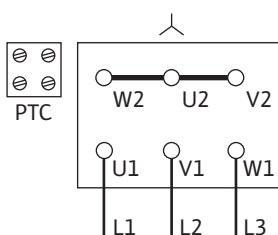
Fig. 13: Y-свързване
