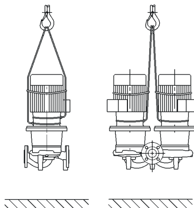
Fig. 1: Транспортиране на помпата
