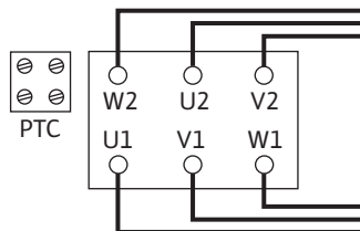
Fig. 14: Y-Δ-свързване
