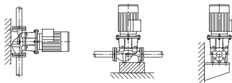
Fig. 4: Изглед IPL – монтиране върху фундамент (≤ 7,5 kW)
