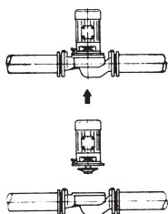
Fig. 3: Изглед IPL – тръбен монтаж
