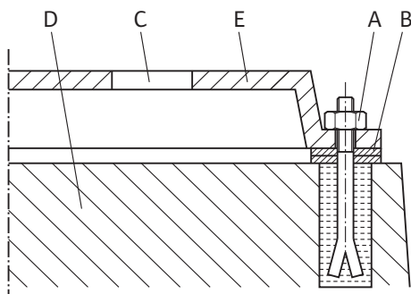
Fig. 9: Пример за закрепване към фундамент с холендър
