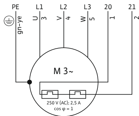
Fig. 7: 3~电机接线图
