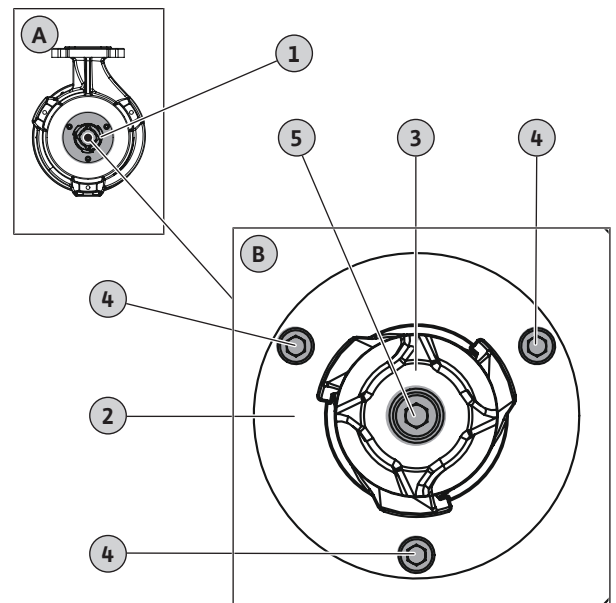
Fig. 9: 更换切碎机
