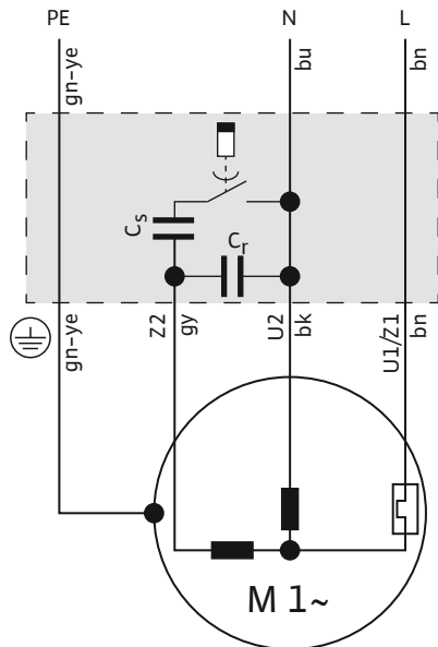
Fig. 6: 1~电机接线图
