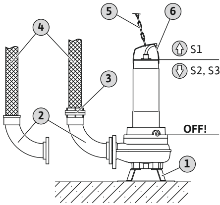
Fig. 5: 移动湿井安装
