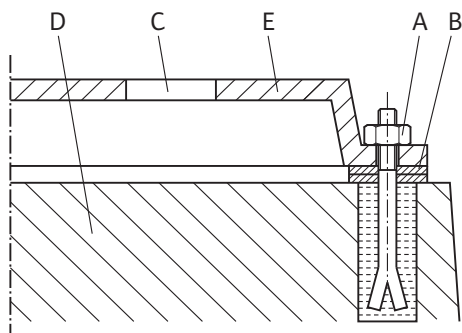
Fig. 12: Eksempel på en fundamentforskrumning
