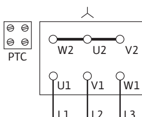
Fig. 15: Couplage Y
