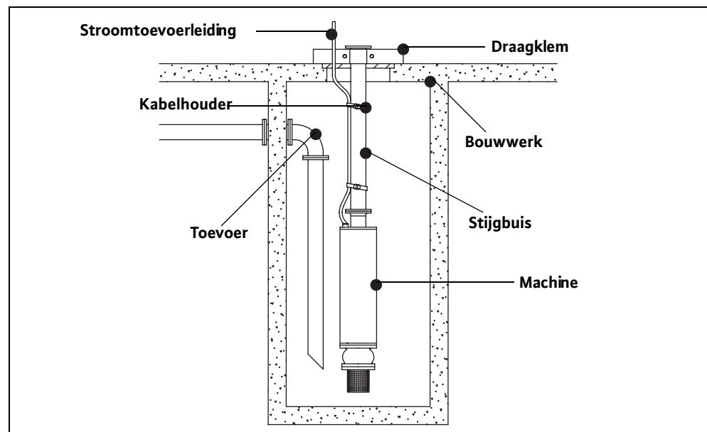
Afb. 5-3: Gestandaardiseerde uitvoering – horizontale inbouw
