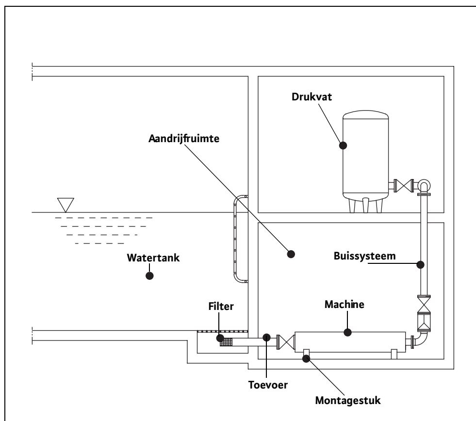
Afb. 5-2: Verticale inbouw
