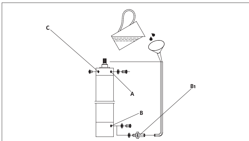
Рис. С-1: Заполнение двигателя
