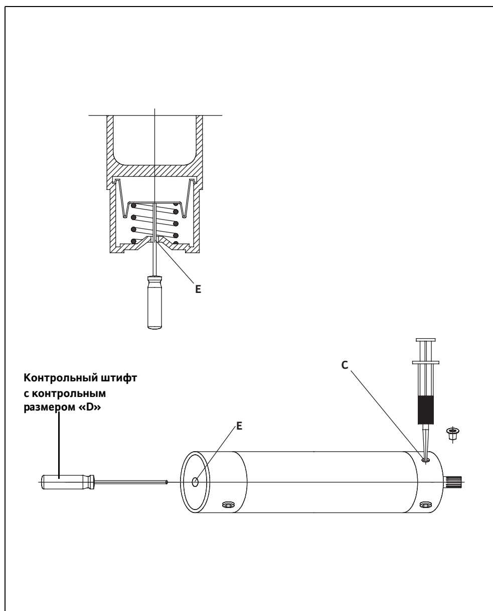
Рис. С-2: Контроль и коррекцию уровня заполнения
