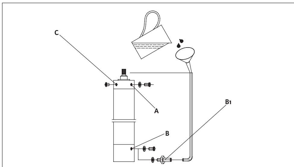
Фиг. С-1: Запълване на мотора
