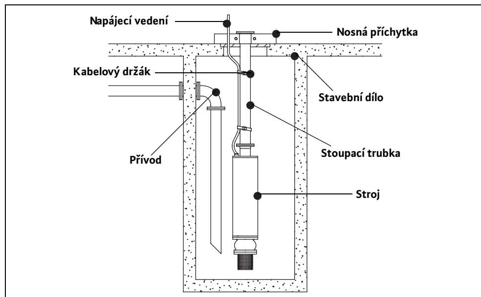
Obr. 5-1: Příklad vestavby
