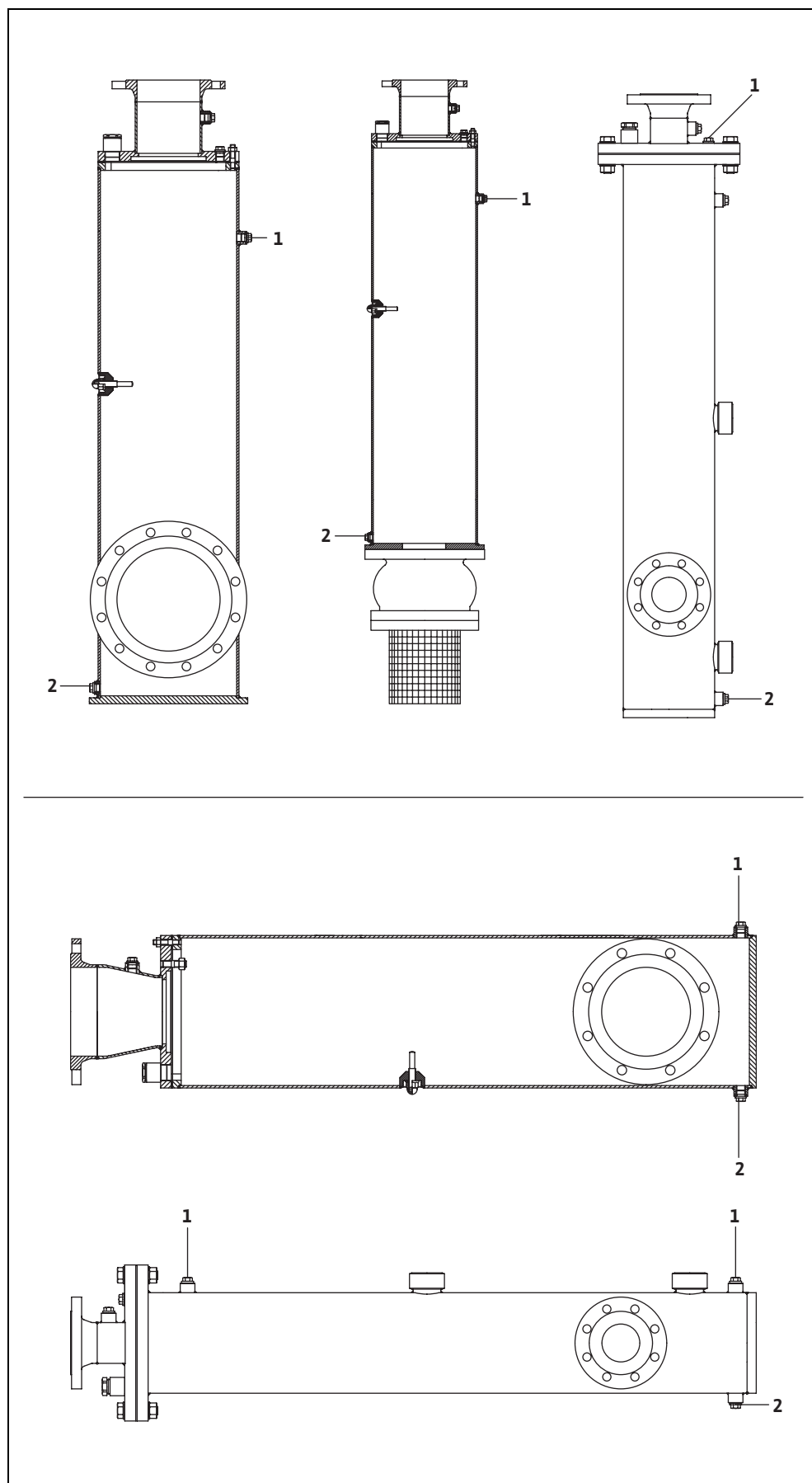
Obr. 5-2: Příklad vestavby
