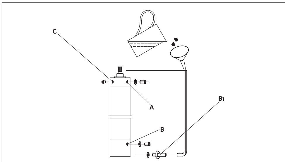
Abb. C-1: Motor befüllen
