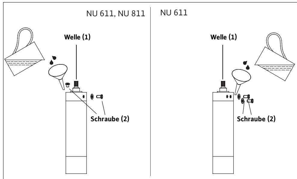
Abb. D-1: Motor befüllen
