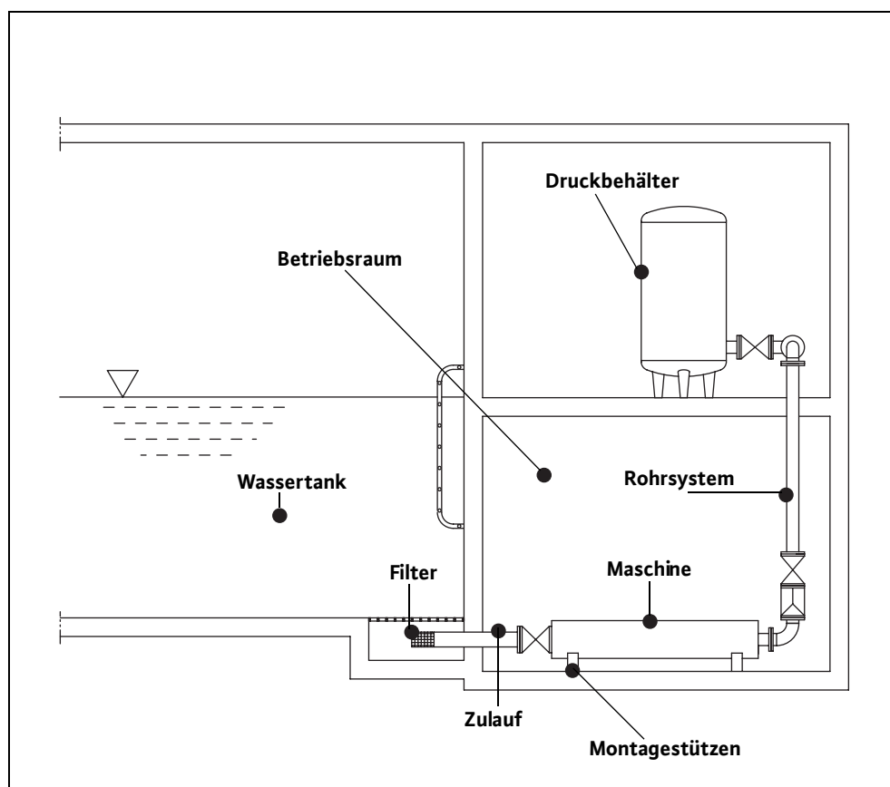
Abb. 5-1: Einbaubeispiel
