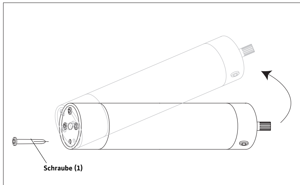
Abb. D-2: Motor entleeren
