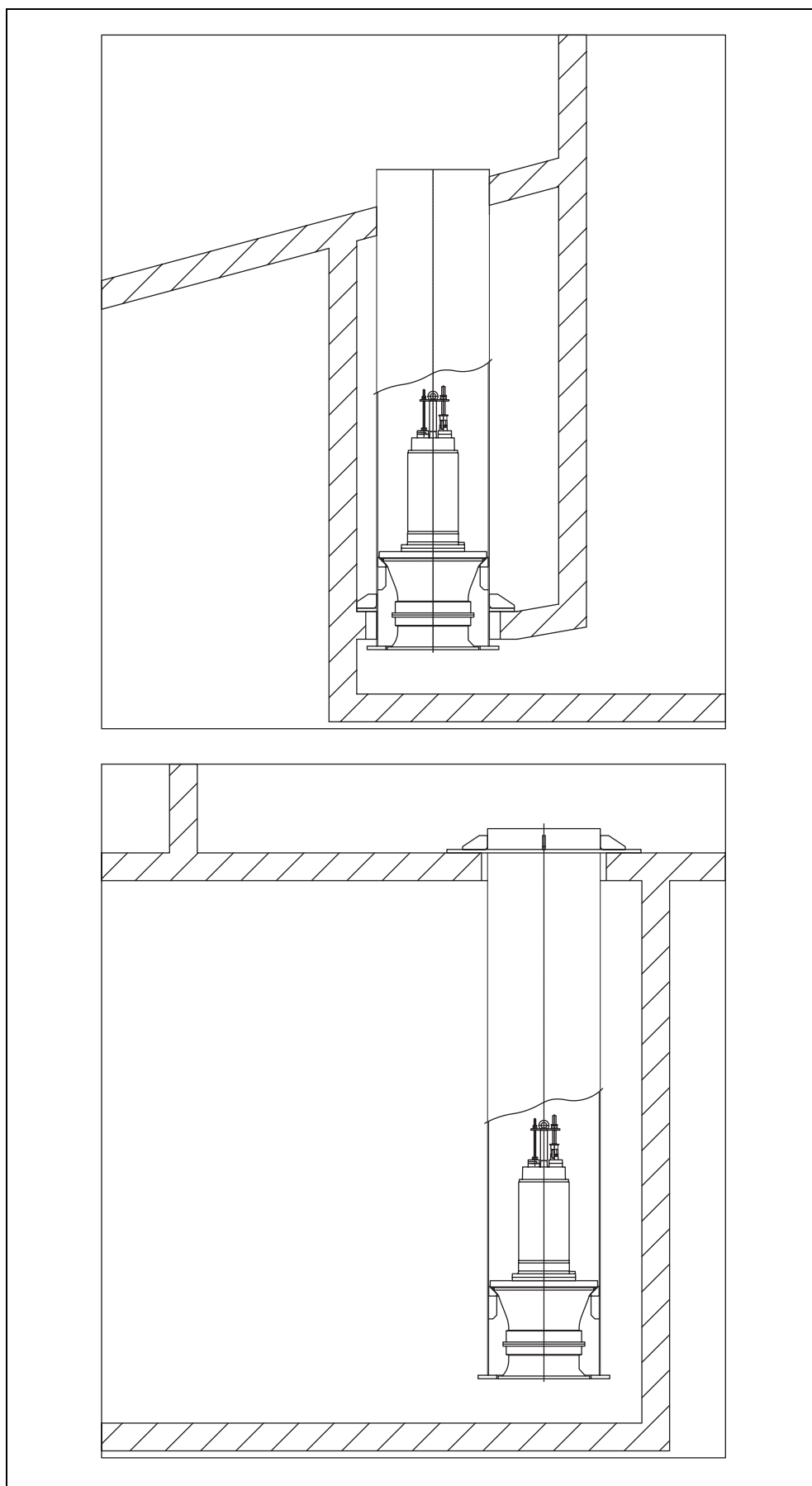
Fig. 5-2: Montare în țeavă, în cameră de admisie acoperită și în evacuare de preaplin în țeavă
