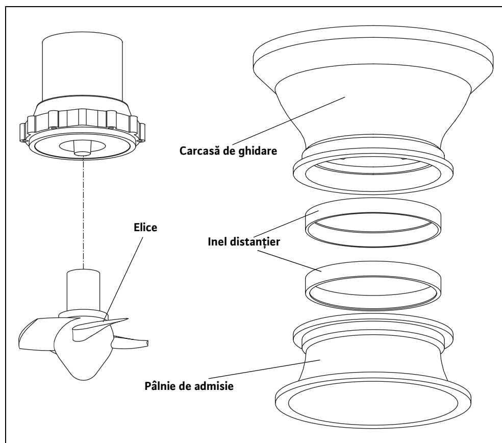
Fig. 3-1: Rotorul elicei
