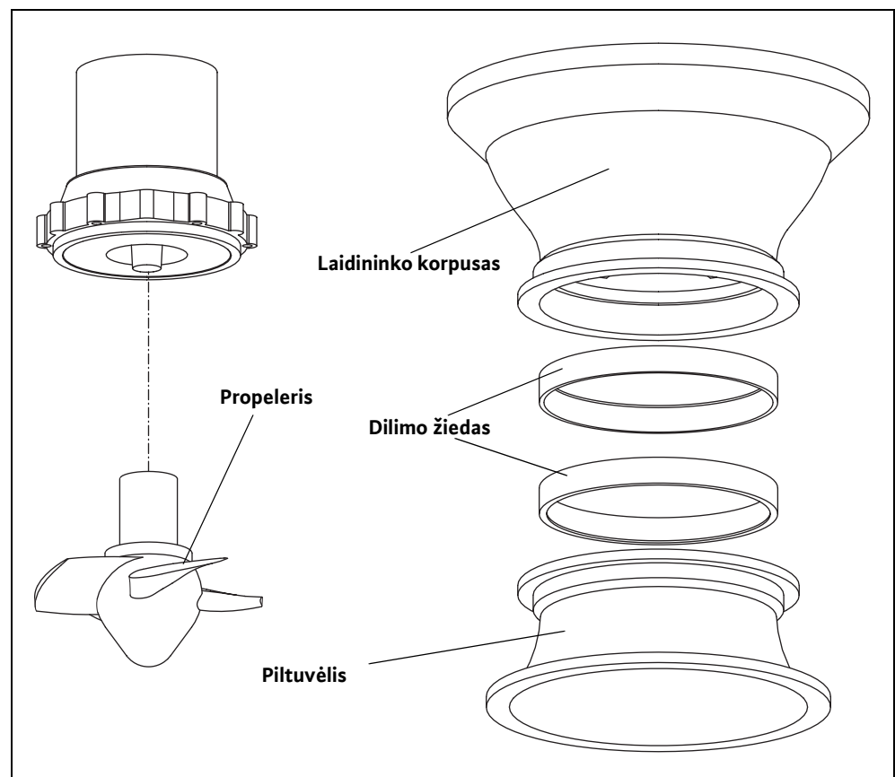
Pav. 3-1: Propelerio ratas
