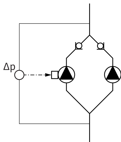
Fig. 9: Exempel – Anslutning differenstrycksgivare i byröransvändning
