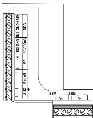
Fig. 26: Styrplintar
