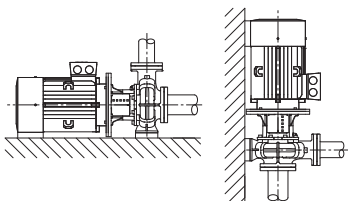
Fig. 4: Vy över Stratos GIGA B
