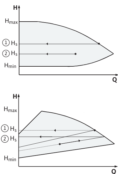
Fig. 32: Reglering \Delta p\text{-}c/\Delta p\text{-}v
