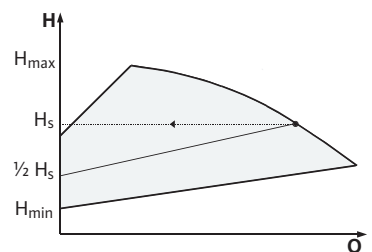
Fig. 7: Reglersätt \Delta p-v
