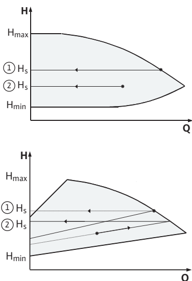
Fig. 32: Регулирование \Delta p -с/ \Delta p -v
