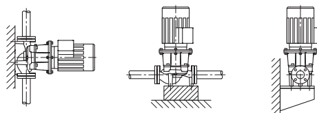
Fig. 3: Вид Stratos GIGA
