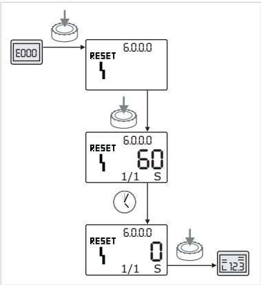
Fig. 51: Квитирование ошибки типа A или D
