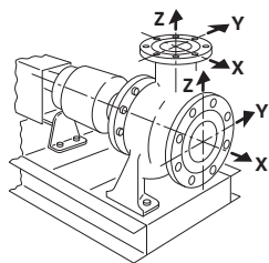
Fig. 22: Случай нагрузки 1A
