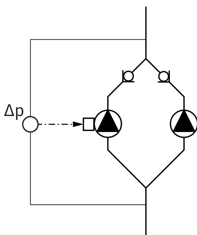
Fig. 9: Пример: подключение дифференциального датчика давления в установке разветвленной трубы
