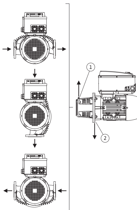
Fig. 14: Допустимые монтажные положения с горизонтальным валом электродвигателя
