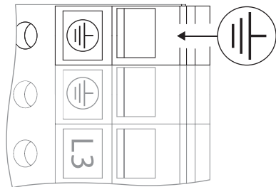
Fig. 28: Дополнительное заземление, мощность двигателя 11 кВт и выше
