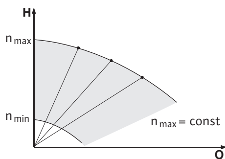
Fig. 8: Tryb sterowania
