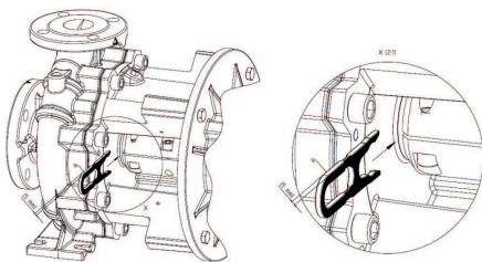
Fig. 47: Zakładanie widełek montażowych
