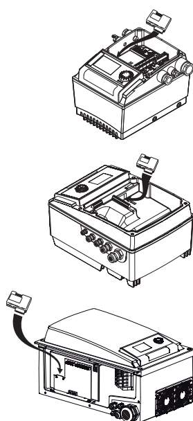
Fig. 10: Wstawić IF-Modul
