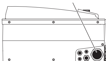
Fig. 24: Dławik przewodu do przewodu zasilającego
