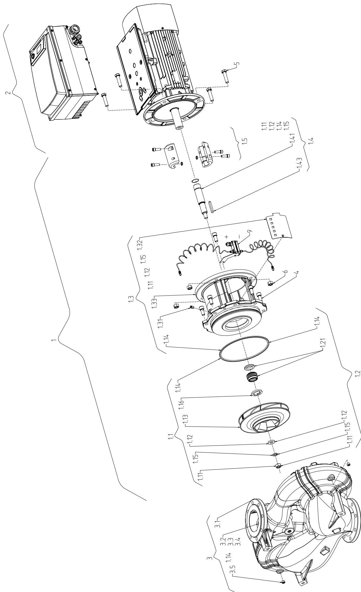
Fig. III: Stratos GIGA-D
