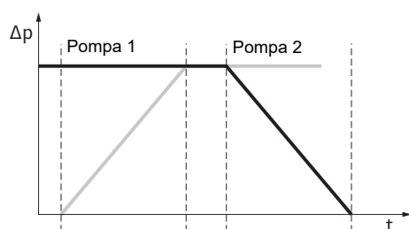
Fig. 11: Zamiana pomp, według schematu
