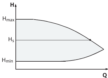
Fig. 6: Säättötapa \Delta p-c
