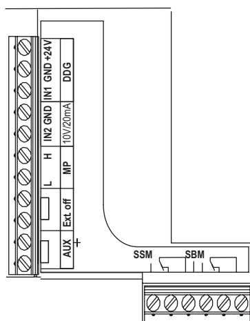
Fig. 26: Ohjausliittimet
