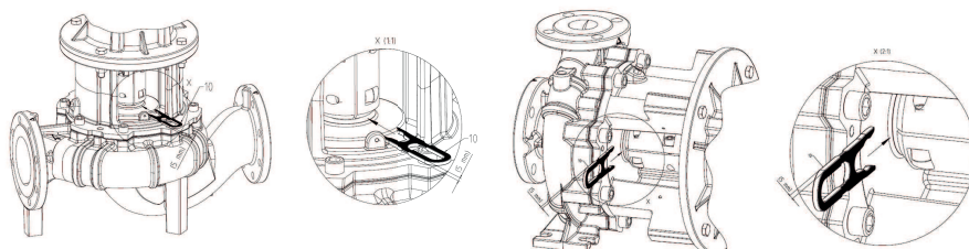
Asennushaarukka säätötöitä varten
