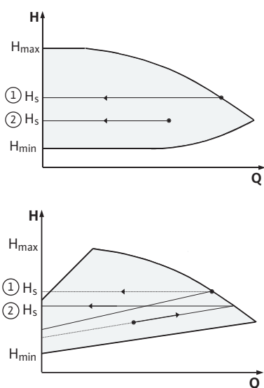
Fig. 32: Säättö \Delta p-c/\Delta p-v
