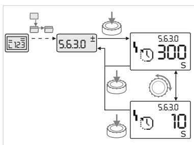
Fig. 44: Säätö ja paluu valikon osaan "Valinta/säädöt"
