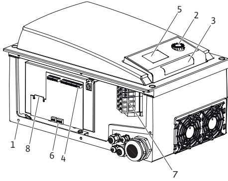
Fig. 5: Elektroniikkamoduuli, yleiskatsaus
