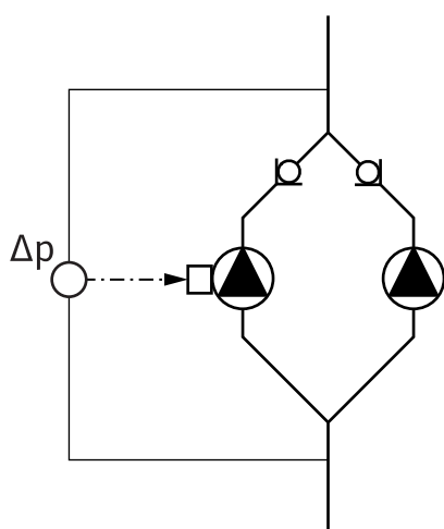
Fig. 9: Esimerkki – paine-eroanturin liittäminen Y-putkiasennuksessa
