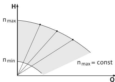
Fig. 8: Manuaalinen säätökäyttö
