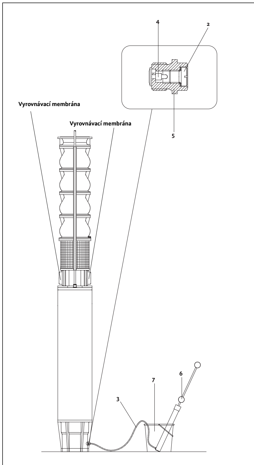
Obr. H-1: Plnění konstrukční řady U21...
