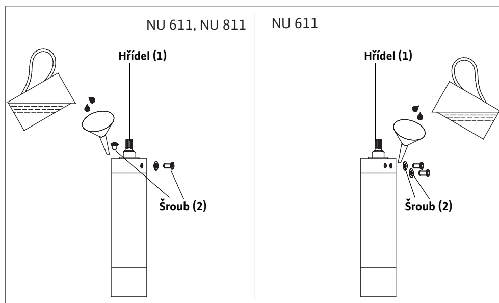
Obr. E-1: Plnění motoru
