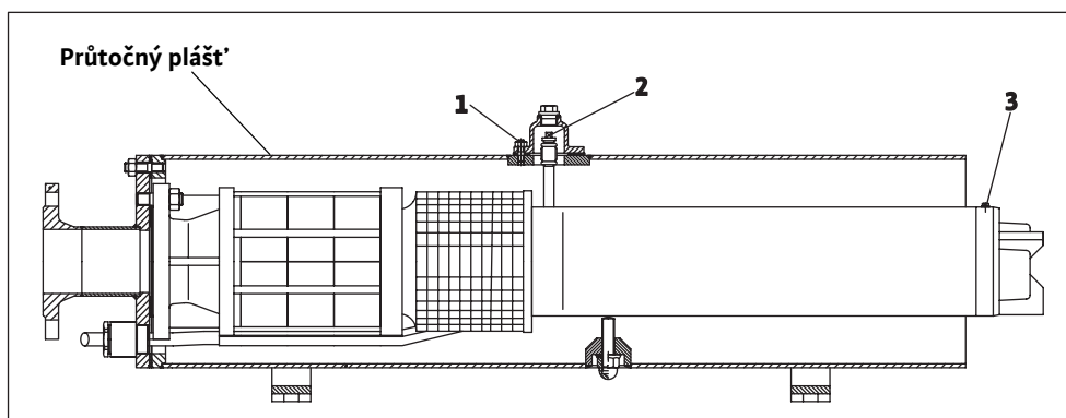
Obr. I-1: Průtočný plášť horizontální, plnění bez demontáže
