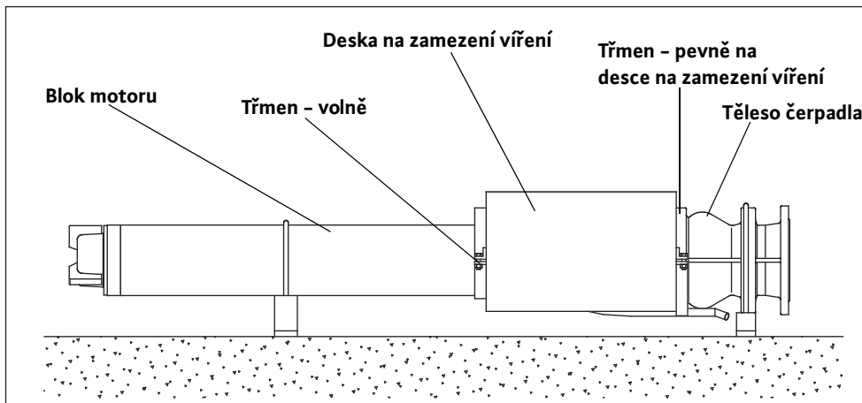
Obr. C-1: Montáž / demontáž desky na zamezení víření
