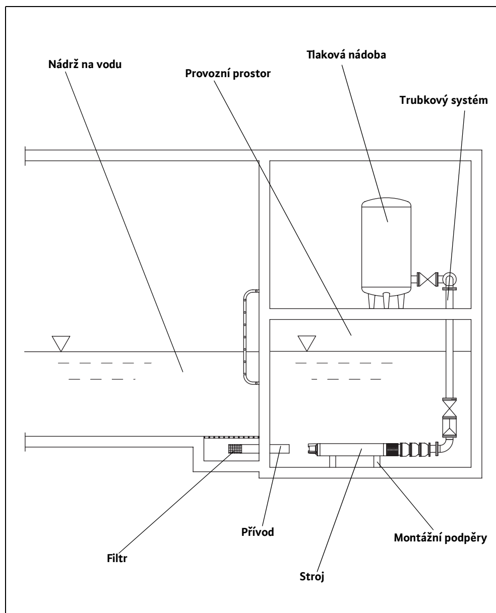
Obr. 5-4: Horizontální montáž do čerpacího zařízení
