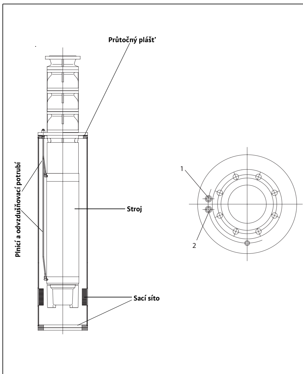
Obr. I-3: Průtočný plášť vertikální, plnění bez demontáže
