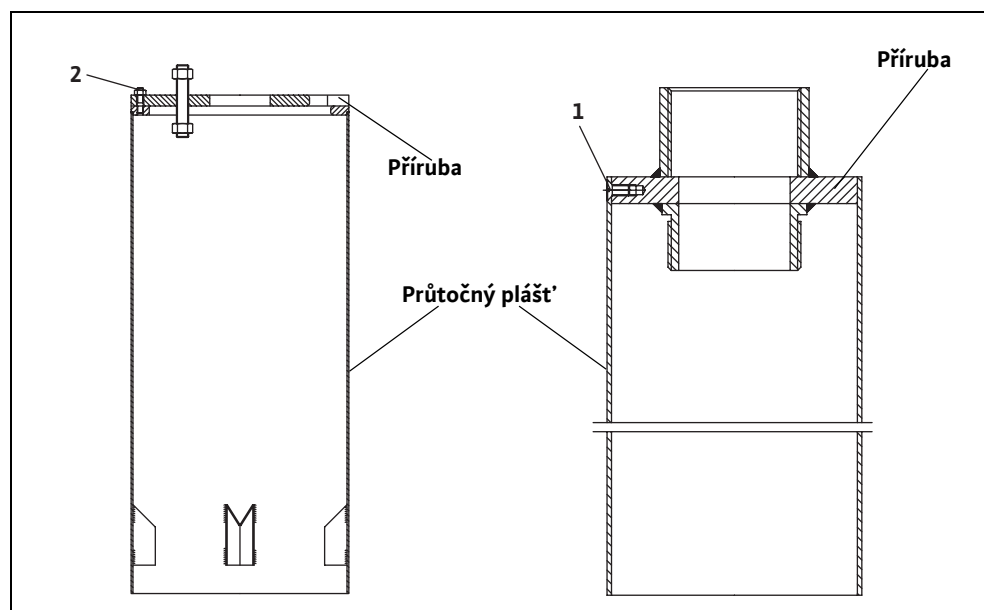
Obr. I-2: Průtočný plášť vertikálně, plnění po demontáži
