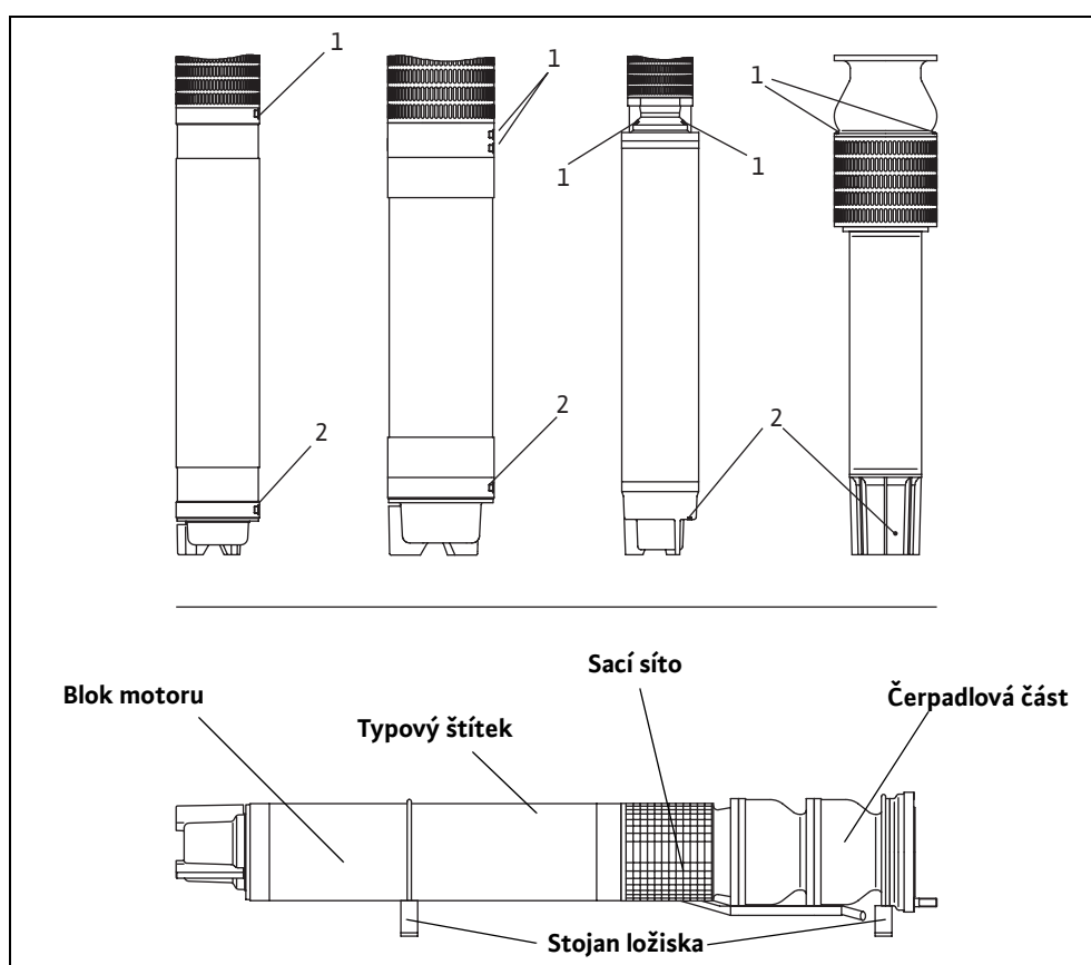
Obr. 5-1: Kontrola a doplnění náplně motoru- vertikální a horizontální montáž
