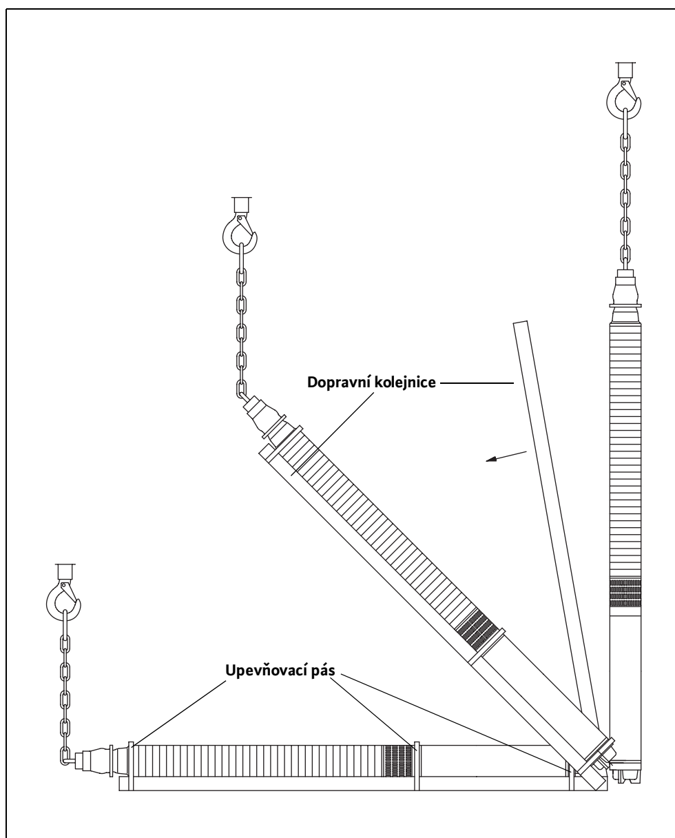
Obr. G-1: Dlouhý stroj s dopravní kolejnicí
