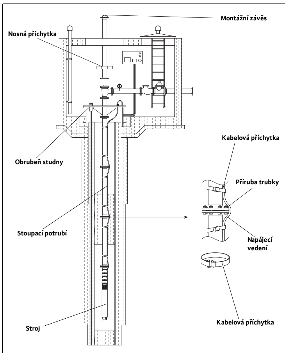
Obr. 5-2: Vertikální montáž
