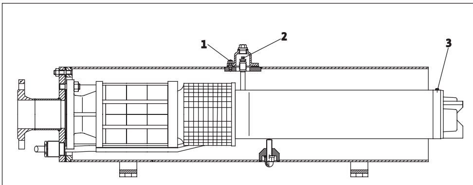
Şekil I-1: Yatay su ceketinin sökülmeden doldurulması
