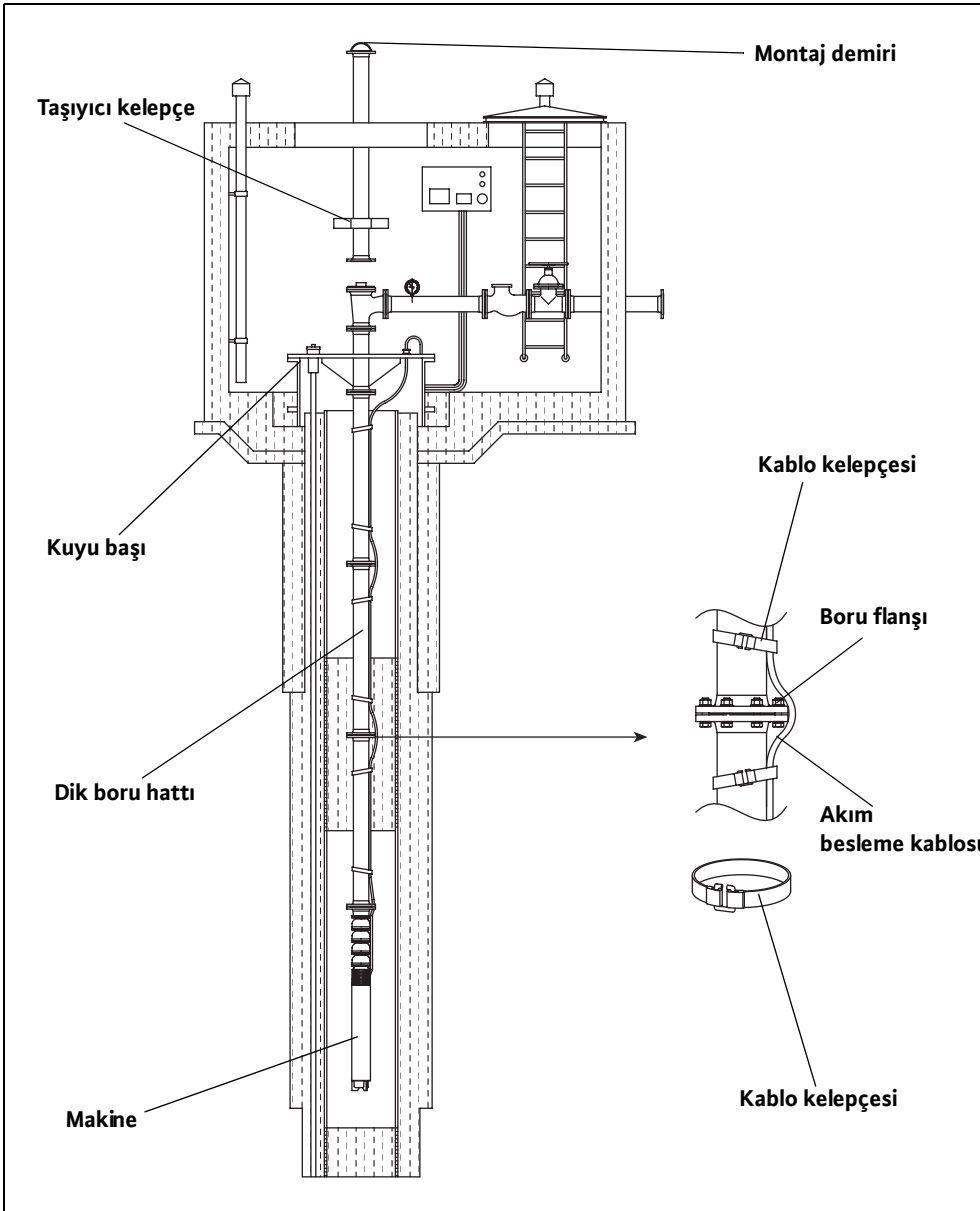
Şekil. 5-2: Düşey montaj
