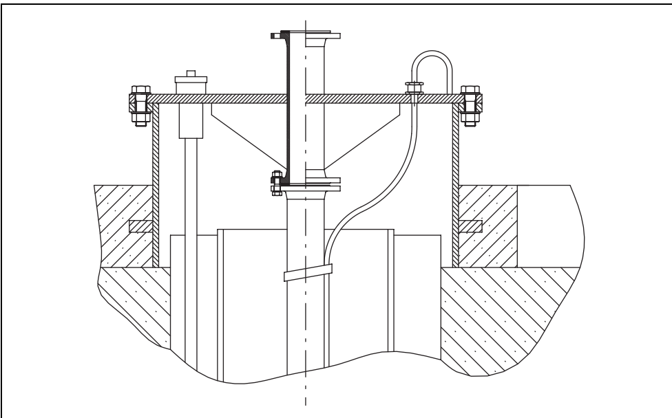
Şekil. 5-3: Kuyu başı
