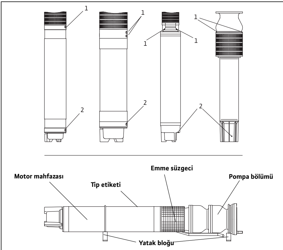
Şekil 5-1: Motor dolumunun kontrolü ve doldurulması - düsey ve yatay montaj
