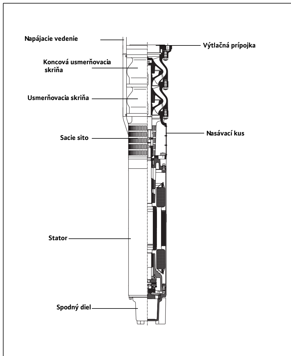
Obr. 3-1: Konštrukcia stroja
