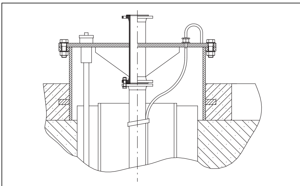
Obr. 5-3: Obruba studne
