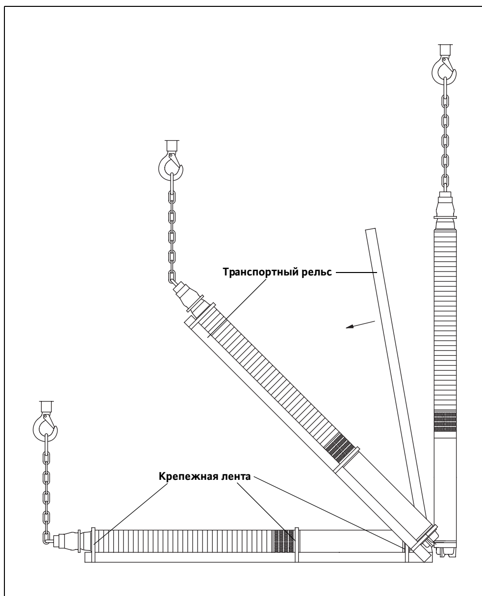
Рис. G-1: Длинное оборудование на транспортном рельсе
