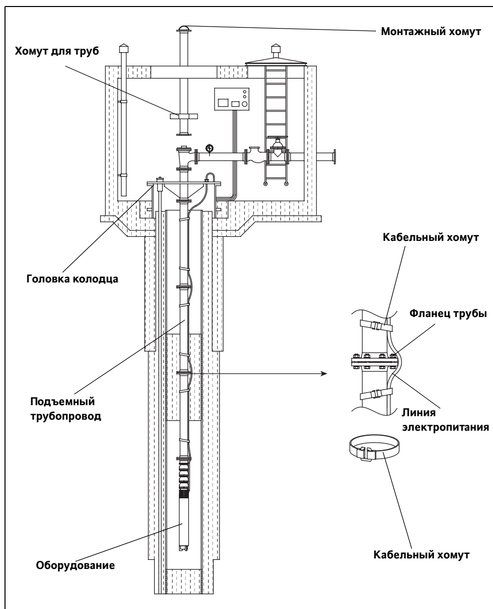
Рис. 5-2: Вертикальный монтаж
