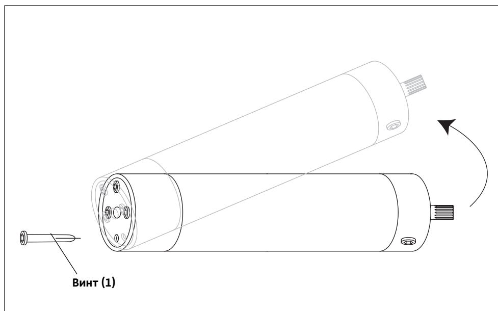
Рис. Е-2: Опорожнение двигателя
