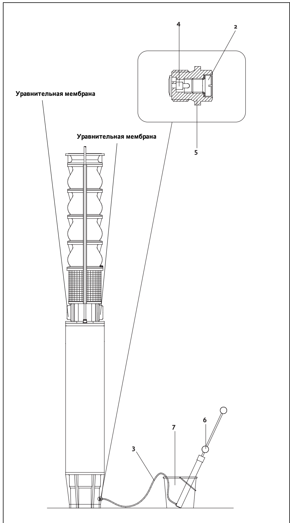
Рис. Н-1: Заливка двигателей ряда U21...
