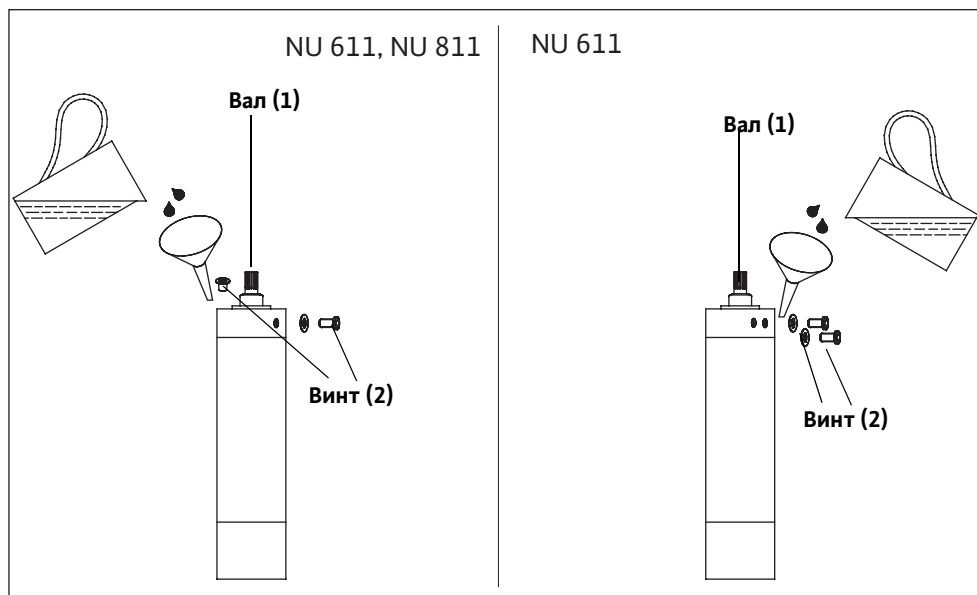
Рис. Е-1: Заполнение двигателя
