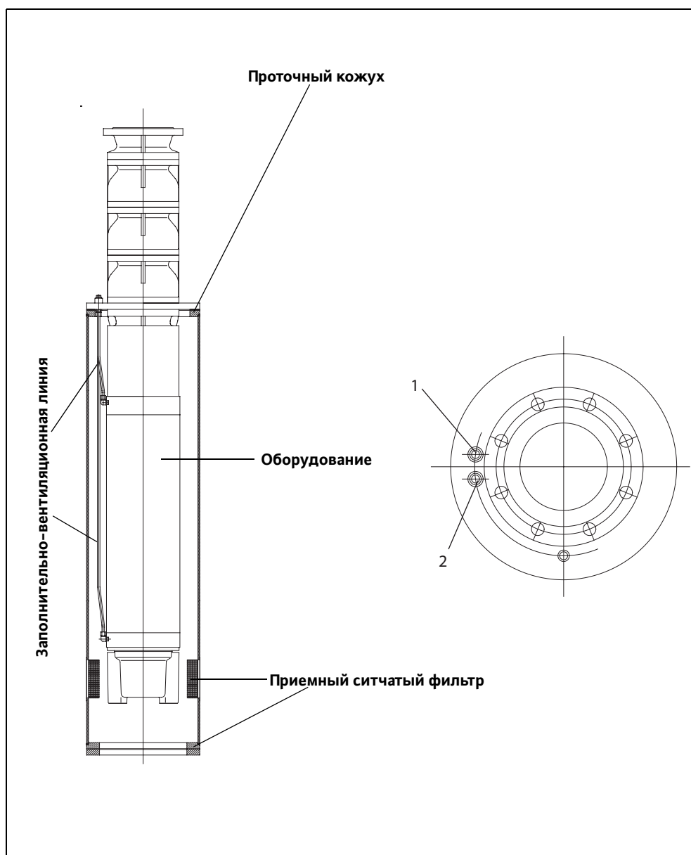
Рис. I-3: Проточный кожух установлен вертикально, заполнение без демонтажа
