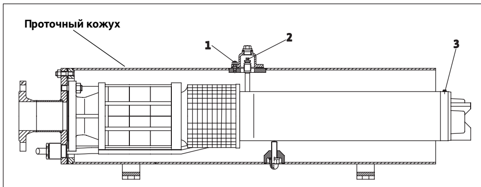
Рис. I-1: Проточный кожух установлен горизонтально, заполнение без демонтажа
