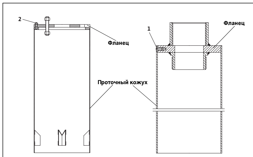
Рис. I-2: Проточный кожух установлен вертикально, заполнение после демонтажа
