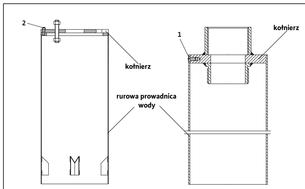
Rys. I-2: Montaż pionowy rurowej przewodnicy wody – napełnianie silnika po demontażu
