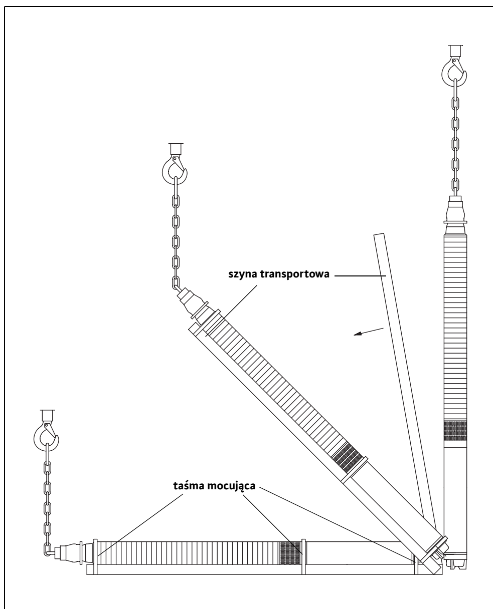
Rys. G-1: Długa pompa z szyną transportową
