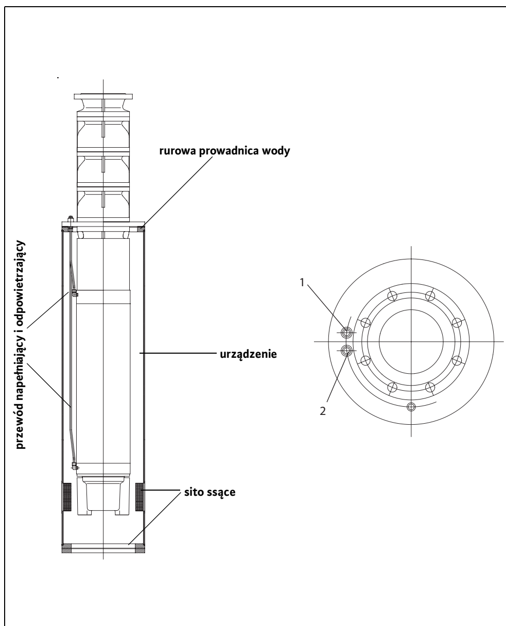
Rys. I-3: Montaż pionowy rurowej przewodnicy wody – napełnianie silnika bez demontażu
