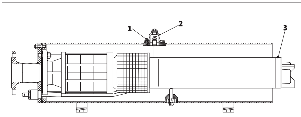
Rys. I-1: Montaż poziomy rurowej przewodnicy wody – napełnianie bez demontażu
