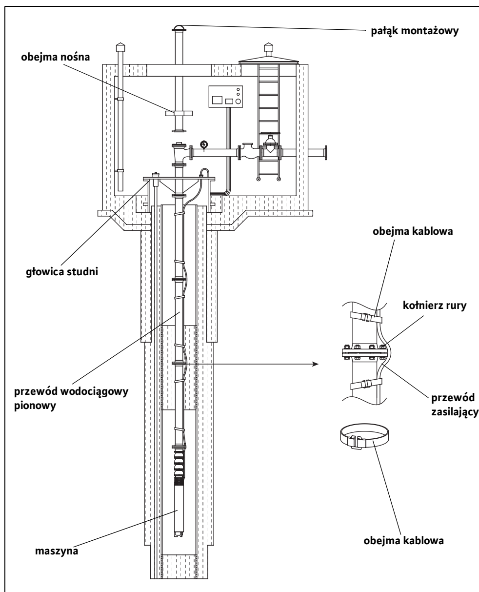
Rys. 5-2: Zabudowa pionowa
