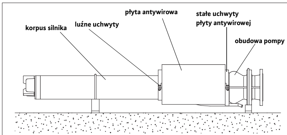
Rys. C-1: Montaż / demontaż płyty antywirowej
