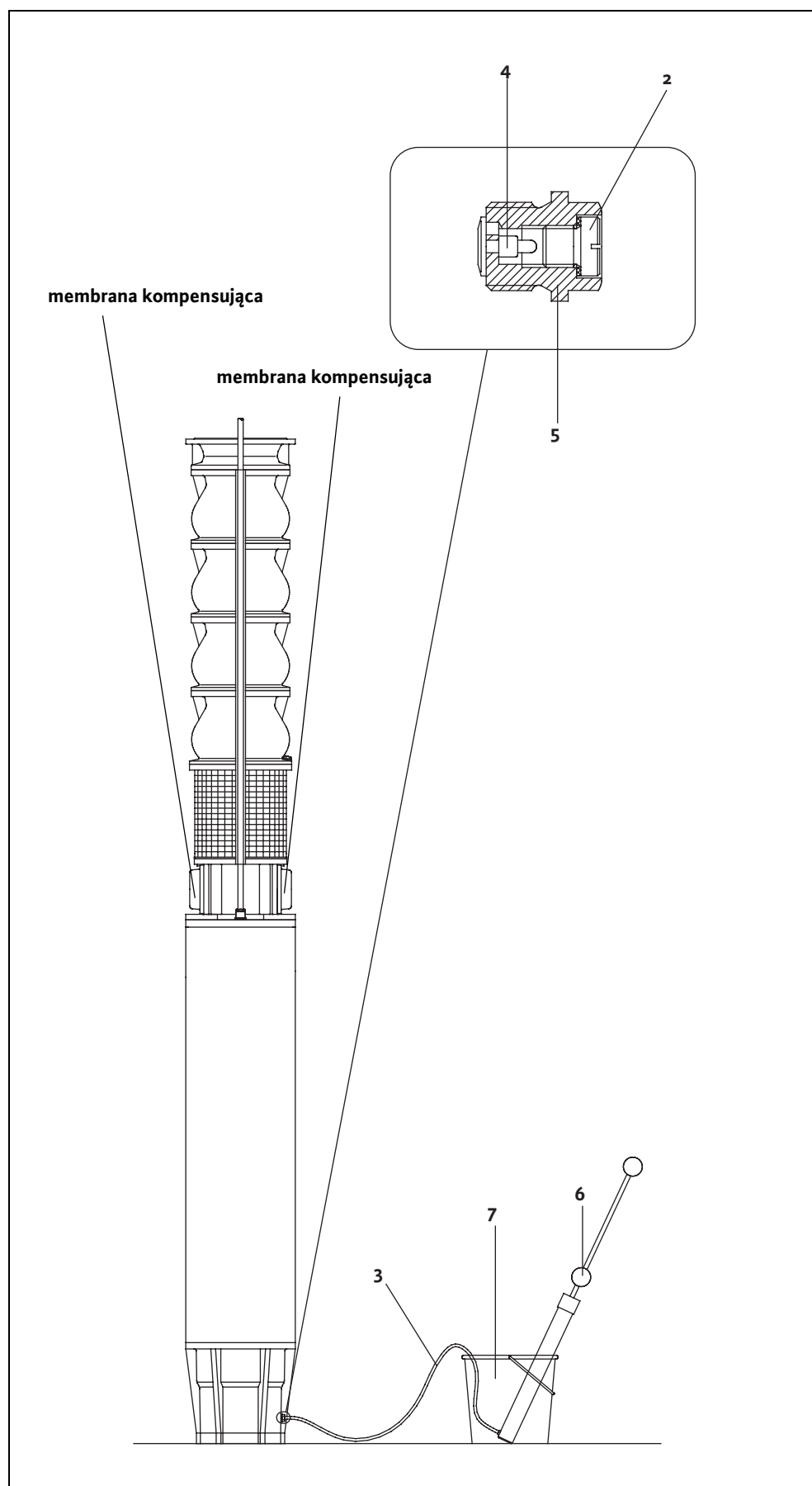
Rys. H-1: Napełnianie silników wersji U21...
