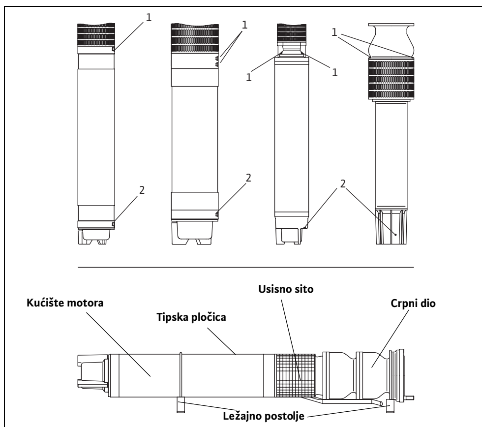
Sl. 5-1: Kontrola i dolijevanje motornog punila – okomita i vodoravna ugradnja
