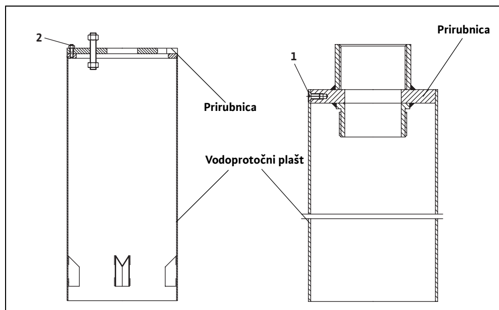
Sl. I-2: Vodoprotocni plašt je okomit, puniti nakon demontaže
