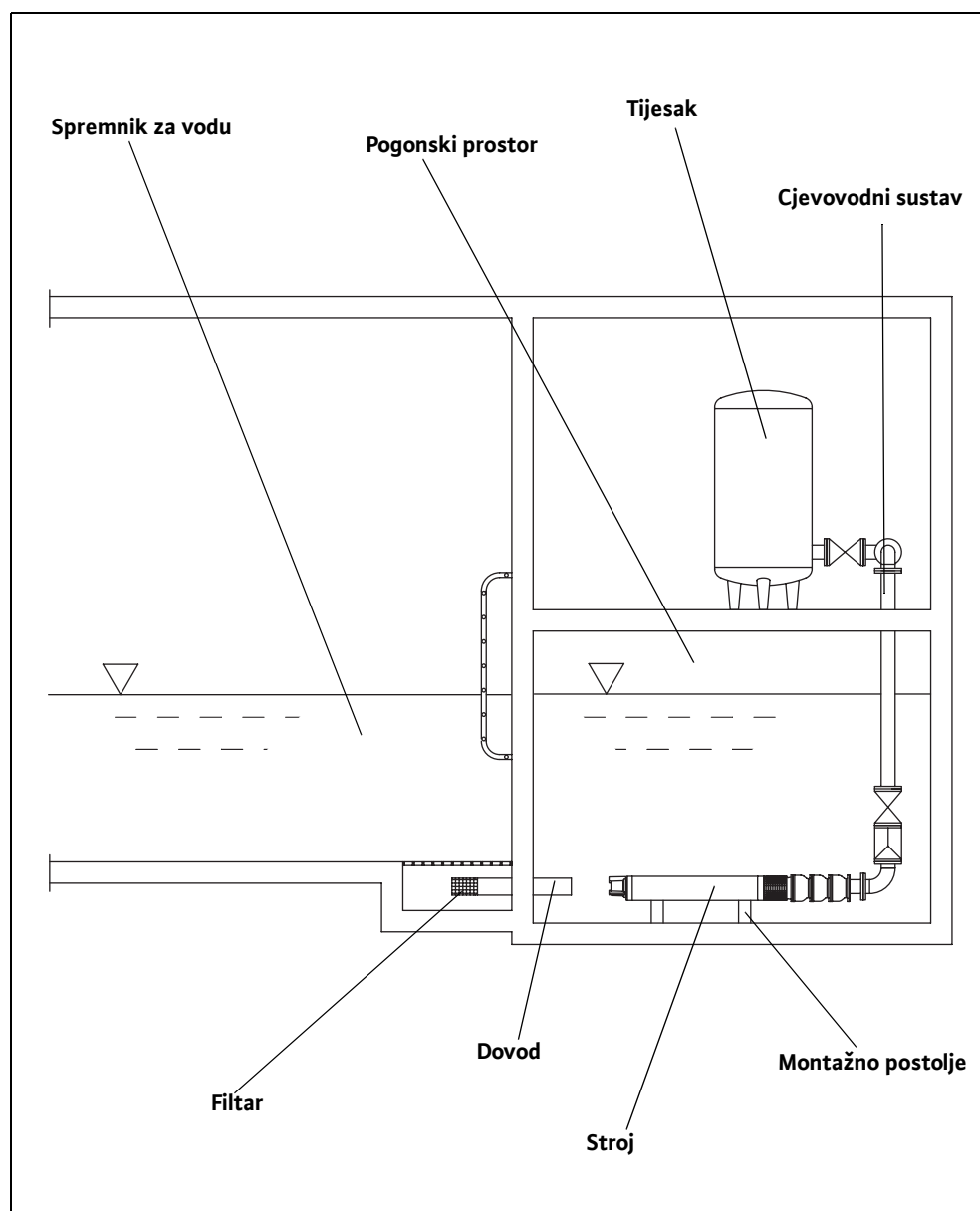
Sl. 5-4: Vodoravna ugradnja u crpnu postaju
