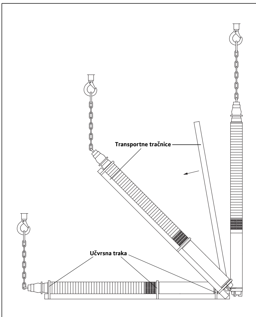
Sl. G-1: Dugački stroj s transportnim tračnicama
