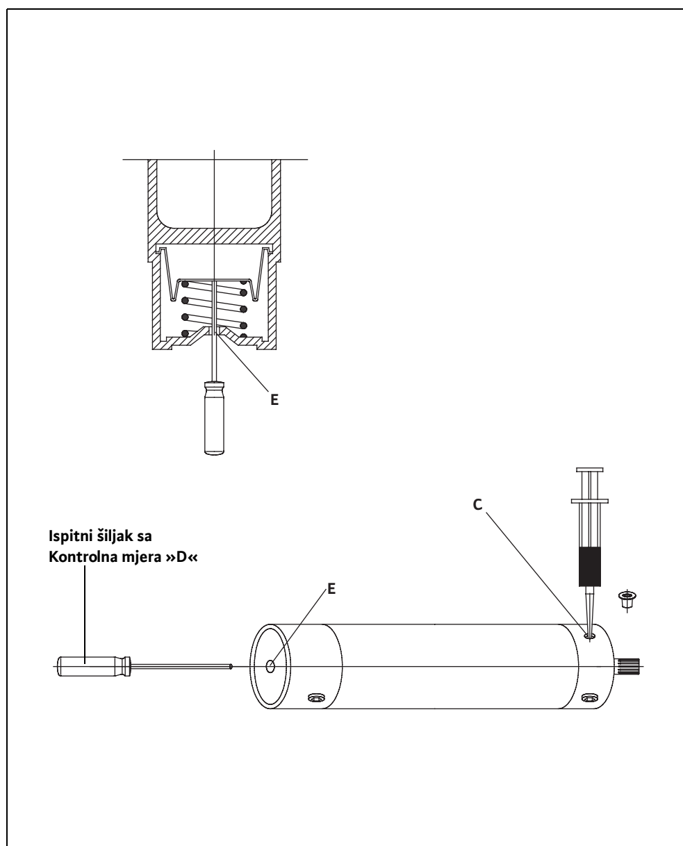
Sl. D-2: Provjera razine i korekcija
