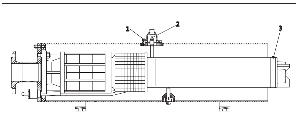
Sl. I-1: Vodoprotlačni plašt vodoravan, punjenje bez demontaže
