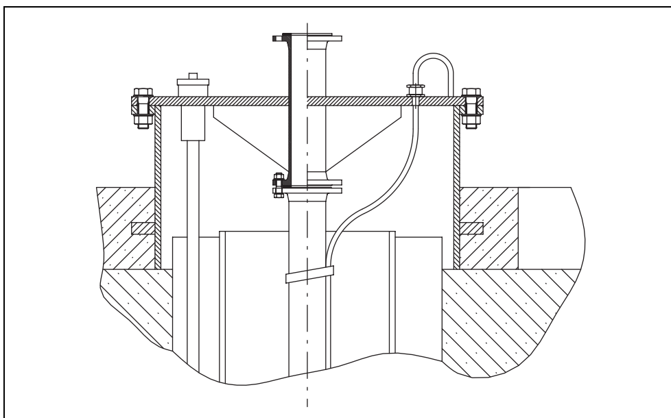
Sl. 5-3: Glava bunara
