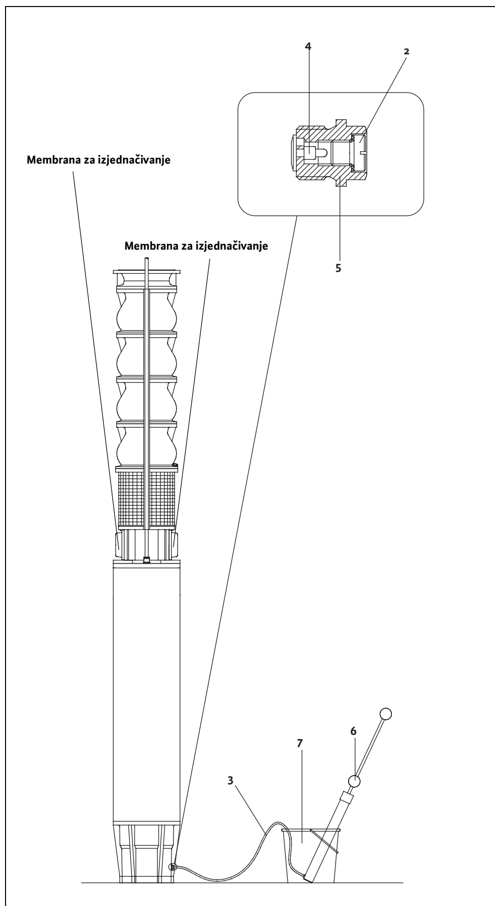
Sl. H-1: Dopunjavanje izvedbene serije U21...
