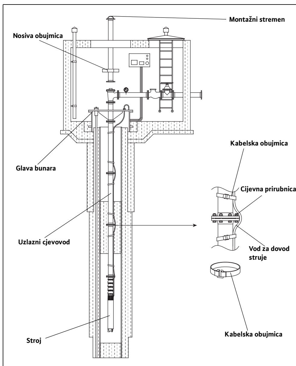
Sl. 5-2: Okomita ugradnja
