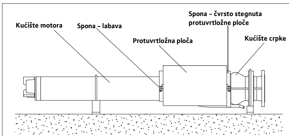
Sl. C-1: Montaža / demontaža protuvrtložne ploče
