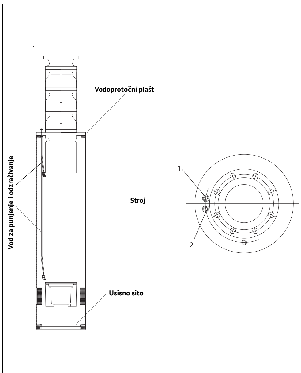
Sl. I-3: Vodoprotlačni plašt je okomit, puniti bez demontaže
