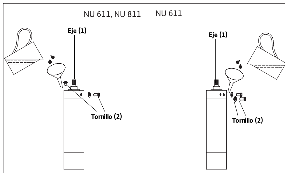
Fig. E-1: Llenar el motor
