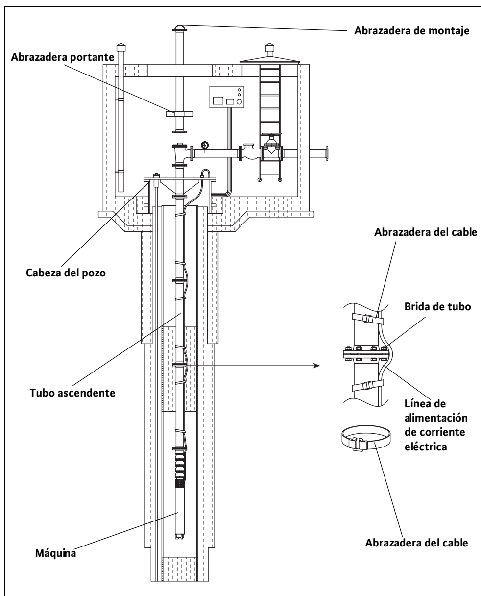
Fig. 5-2: Montaje vertical
