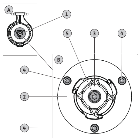
Fig. 9: Byte av skärverk
