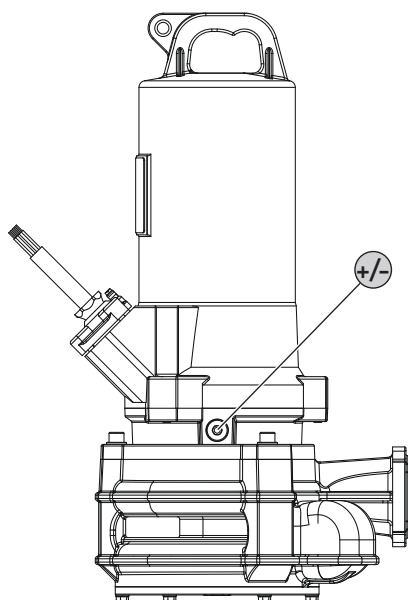
Fig. 8: Tätningskammare: Oljebyte
