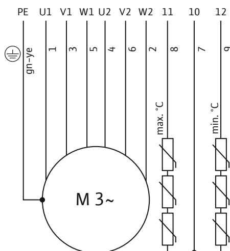
Fig. 7: Anslutningsschema 3~-motor: Stjärntriangelstart, PTC-sensor
