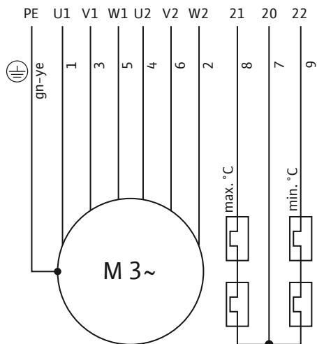
Fig. 6: Anslutningsschema 3~-motor: Stjärntriangelstart, bimetallsensor
