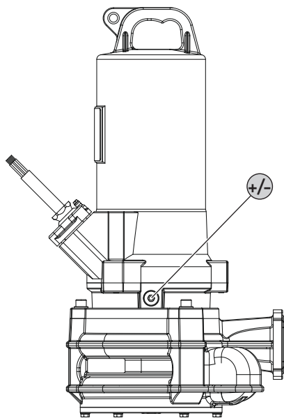
Fig. 8: Tesnilna komora: Menjava olja
