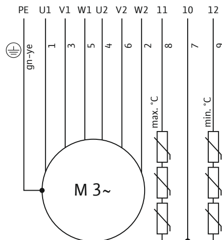
Fig. 7: Priključni načrt 3~–motor: Vkllop zvezda – trikot, tipalo PTC
