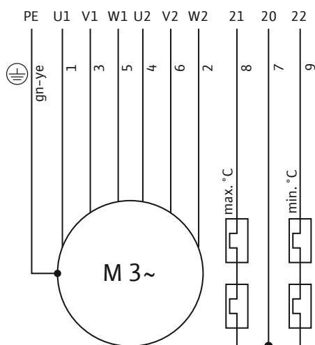
Fig. 6: Priključni načrt 3~-motor: Vklon zvezda – trikot, bimetalno tipalo
