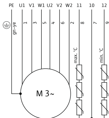
Fig. 7: Schéma pripojenia 3~motor: Rozbeh hviezda-trojuholník, snímač PTC
