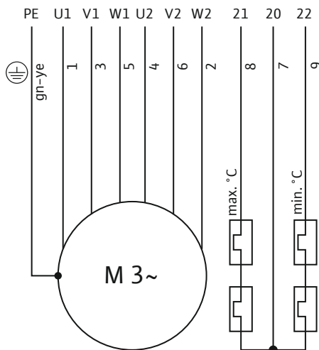
Fig. 6: Schéma pripojenia 3~motor: Rozbeh hviezda–trojuholník, bimetalový pás
