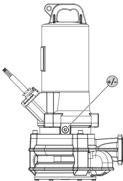
Fig. 8: Câmara de vedação: Mudança de óleo
