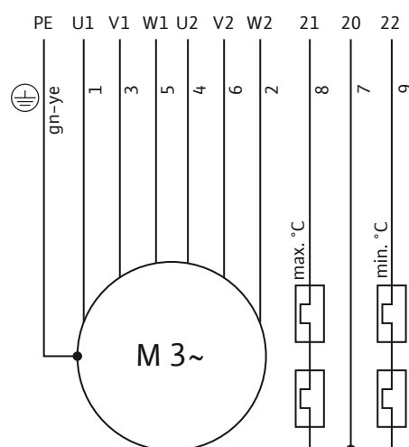
Fig. 6: Esquema de ligações para motor trifásico: Arranque estrela-triângulo, sensor bimetálico
