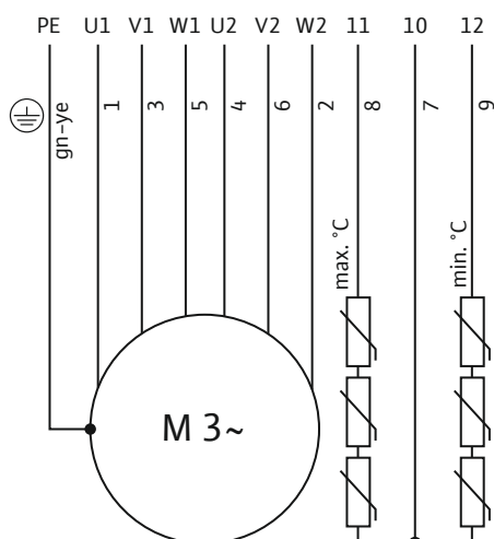
Fig. 7: Esquema de ligações para motor trifásico: Arranque estrela-triângulo, sensor PTC
