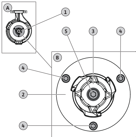
Fig. 9: Substituição do triturador
