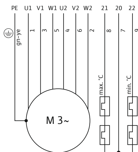
Fig. 6: Aansluitschema 3~-motor: Sterdriehoekstart, bimetaalsensor
