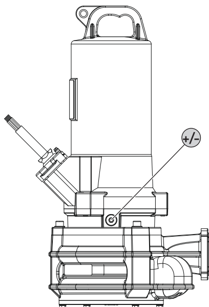
Fig. 8: Afdichtingsruimte: Olieverversen
