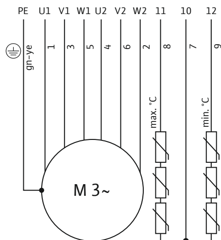
Fig. 7: Aansluitschema 3~-motor: Sterdriehoekinschakeling, PTC-sensor
