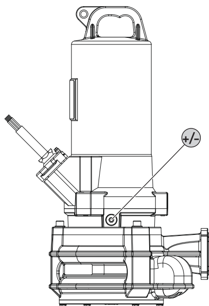
Fig. 8: Blīvēšanas kamera: Eļļas nomaiņa
