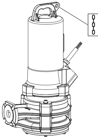
Fig. 1: Anschlagpunkt
