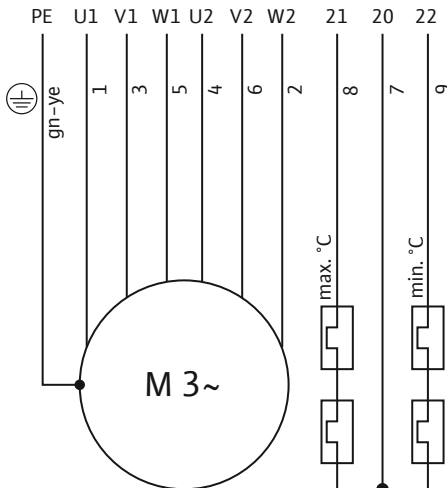
Fig. 6: Anschlussplan 3~-Motor: Stern-Dreieck-Anlauf, Bimetallfühler
