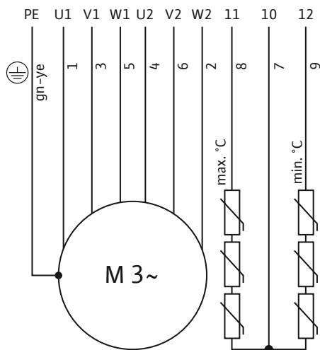
Fig. 7: Anschlussplan 3~-Motor: Stern-Dreieck-Anlauf, PTC-Fühler
