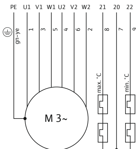
Fig. 6: Esquema de conexión motor 3~: Arranque estrella-triángulo, sensor bimetálico
