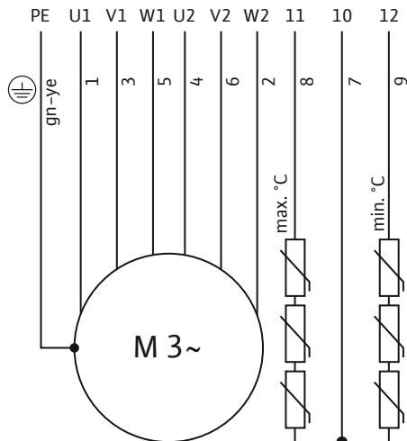
Fig. 7: Esquema de conexión motor 3~: Arranque estrella-triángulo, sensor PTC
