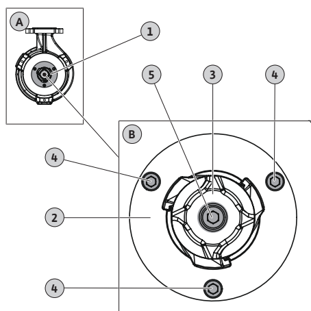
Fig. 9: Αντικατάσταση κοπτήρα
