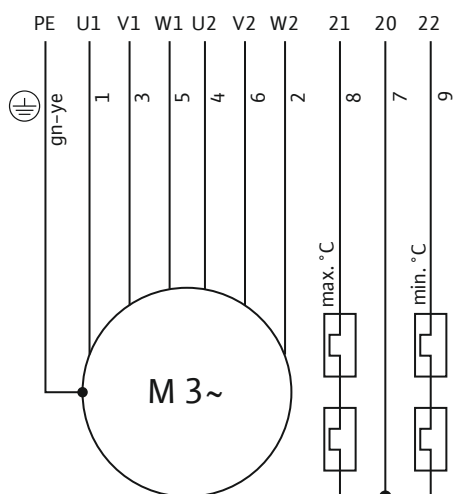
Fig. 6: Σχεδιάγραμμα σύνδεσης 3~ κινητήρας: Ενεργοποίηση αστέρα/τριγώνου, διμεταλλικός αισθητήρας
