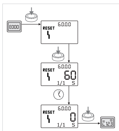
Fig. 53: Validarea tipului de eroare A sau D
