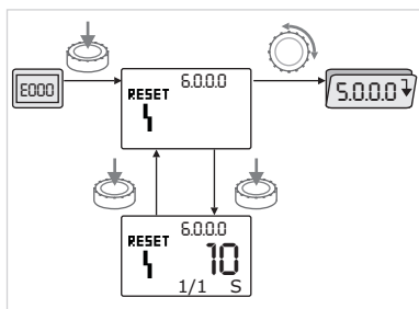
Fig. 50: Navigare în caz de eroare
