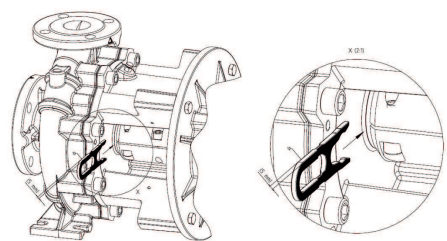
Fig. 47: Atașarea barei de montaj
