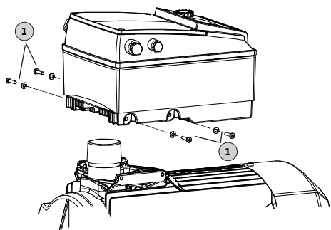
Fig. 49: Conexiunea modul electronic – motor
