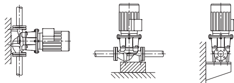
Fig. 3: Vedere IL-E
