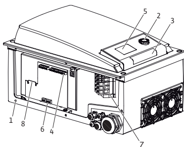
Fig. 5: Prezentare generală a modului electronic
