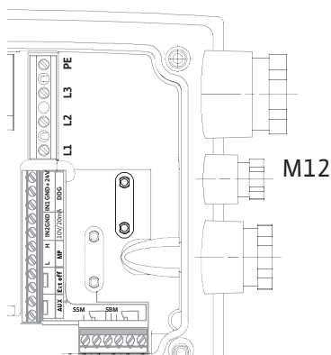
Fig. 25: Conectați ecranul
