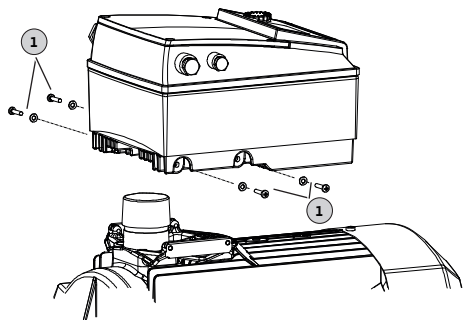
Fig. 48: Înlocuirea modului electronic
