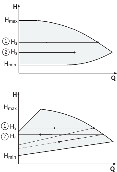
Fig. 32: Reglarea \Delta p\text{-}c/\Delta p\text{-}v
