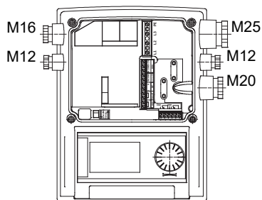
Fig. 29: Presetupe pentru cablu
