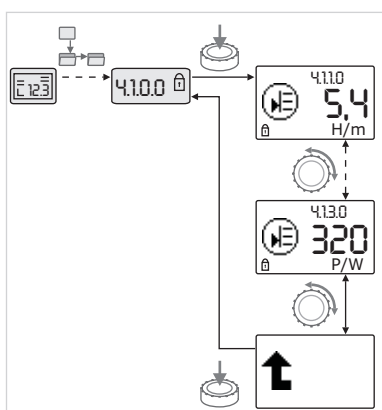
Fig. 46: Accesarea informațiilor
