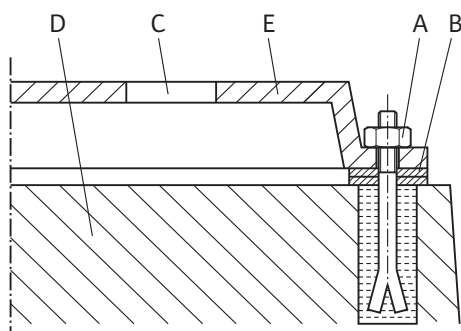
Fig. 16: Exemplu pentru un racord filetat fundație
