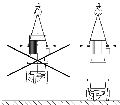
Fig. 2: Transportul motorului
