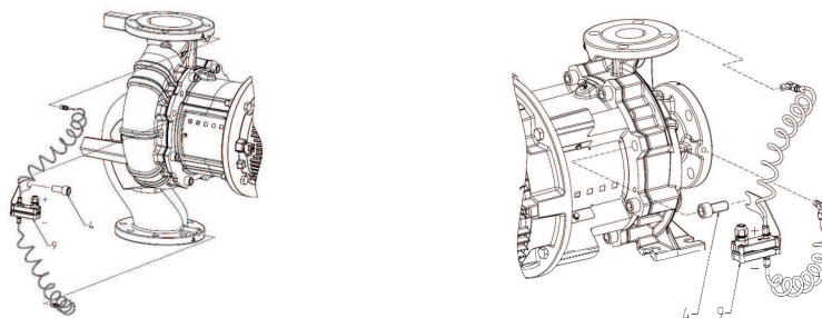
Πίν. 14: Σύνδεση αισθητηρίου διαφορικής πίεσης
