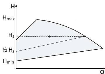
Fig. 7: Είδος ρύθμισης \Delta p-v
