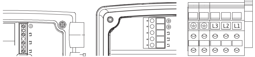
Fig. 27: Ακροδέκτες ισχύος
