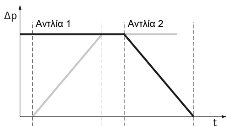
Fig. 11: Εναλλαγή αντλιών, διαγραμματικά
