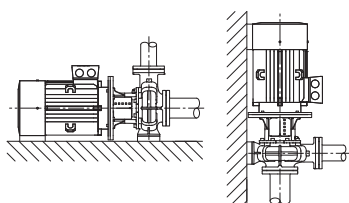
Fig. 4: Όψη Atmos GIGA-B
