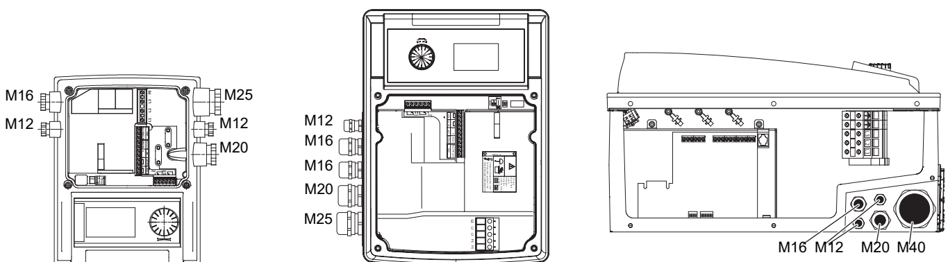
Fig. 29: Στυπιοθλίπτες καλωδίων
