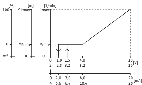
Fig. 12: Χαρακτηριστικά λειτουργίας εισόδων και εξόδων
