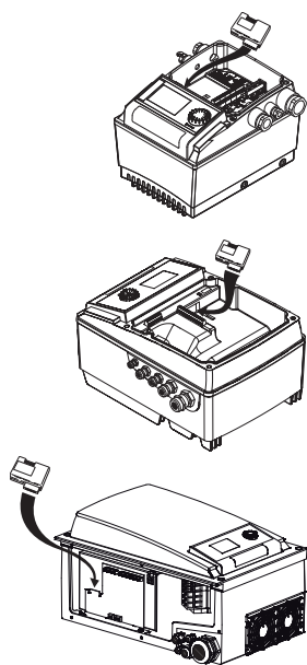
Fig. 10: Χρήση IF-Modul
