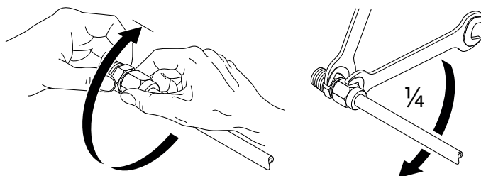
Fig. 19: Περιστρέψτε τη βιδωτή σύνδεση σύσφιξης κατά 1/4
