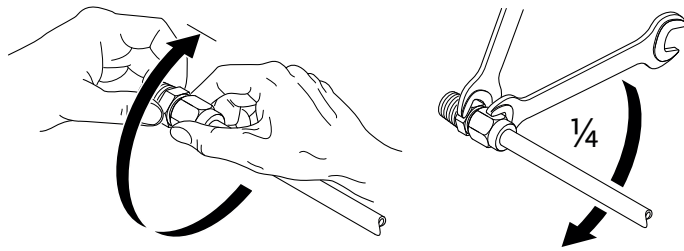
Fig. 19: Dreie klemringskrutilkoblingen 1/4 omdreining til
