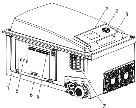
Fig. 5: Elektronikkmodul, oversikt
