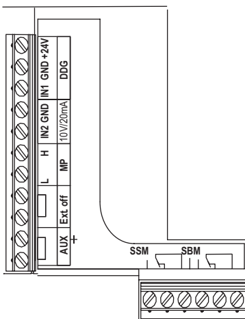
Fig. 26: Kontrollpanel
