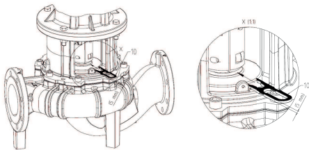
Fig. 47: Plassering av montasjegaффelen
