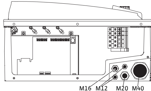
Fig. 29: Kabelskjøter med gjenger
