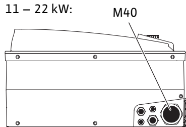
Fig. 24: Kabelskjøt med gjenger for nettilkoblingskabel
