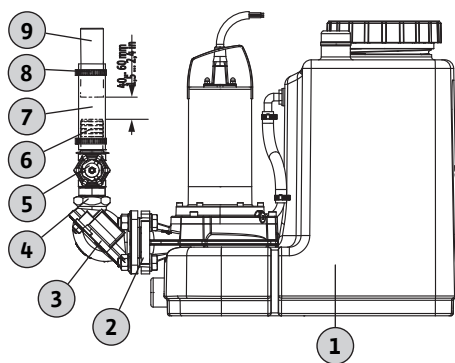
Fig. 3: Druckanschluss anbringen
