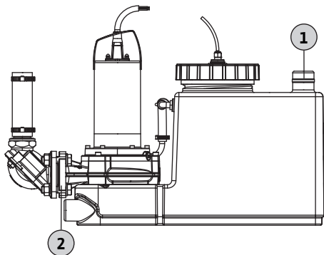
Fig. 6: Raccordo di aerazione e del serbatoio di raccolta
