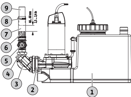
Fig. 3: Montaggio del raccordo di mandata
