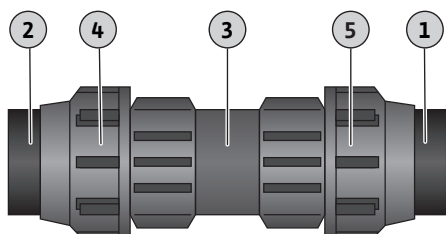
Fig. 6: Racordarea conductei de refulare
