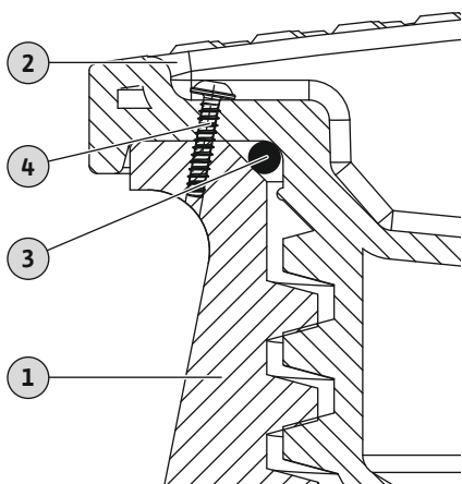
Fig. 17: Instalați și asigurați capacul căminului
