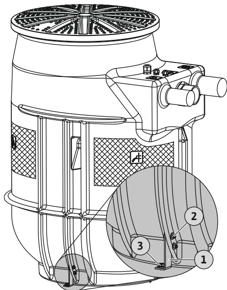
Fig. 3: Amenajarea căminului
