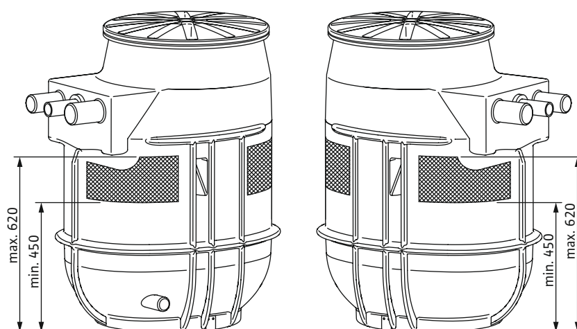
Fig. 8: Suprafețe de alimentare
