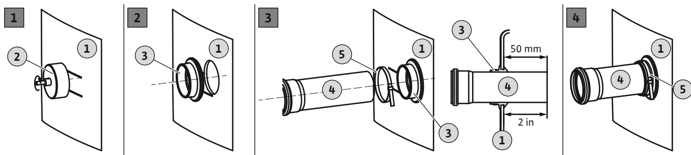
Fig. 9: Racordarea conductei de intrare
