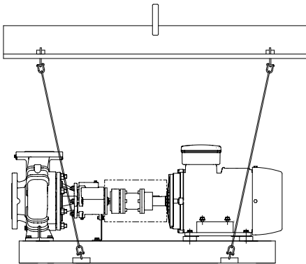
Fig. 2: Aggregat anschlagen
