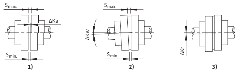
Fig. 11: Kupplungsausrichtung ohne Distanzstück
