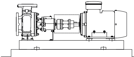
Fig. 5: Fundamentaufstellung des Aggregats
