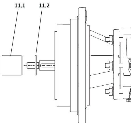
Fig. 21: Gleitlager ausbauen
