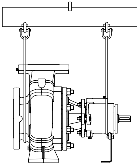
Fig. 1: Pumpe anschlagen
