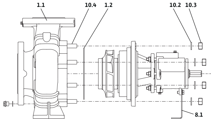
Fig. 19: Einschubeinheit herausziehen
