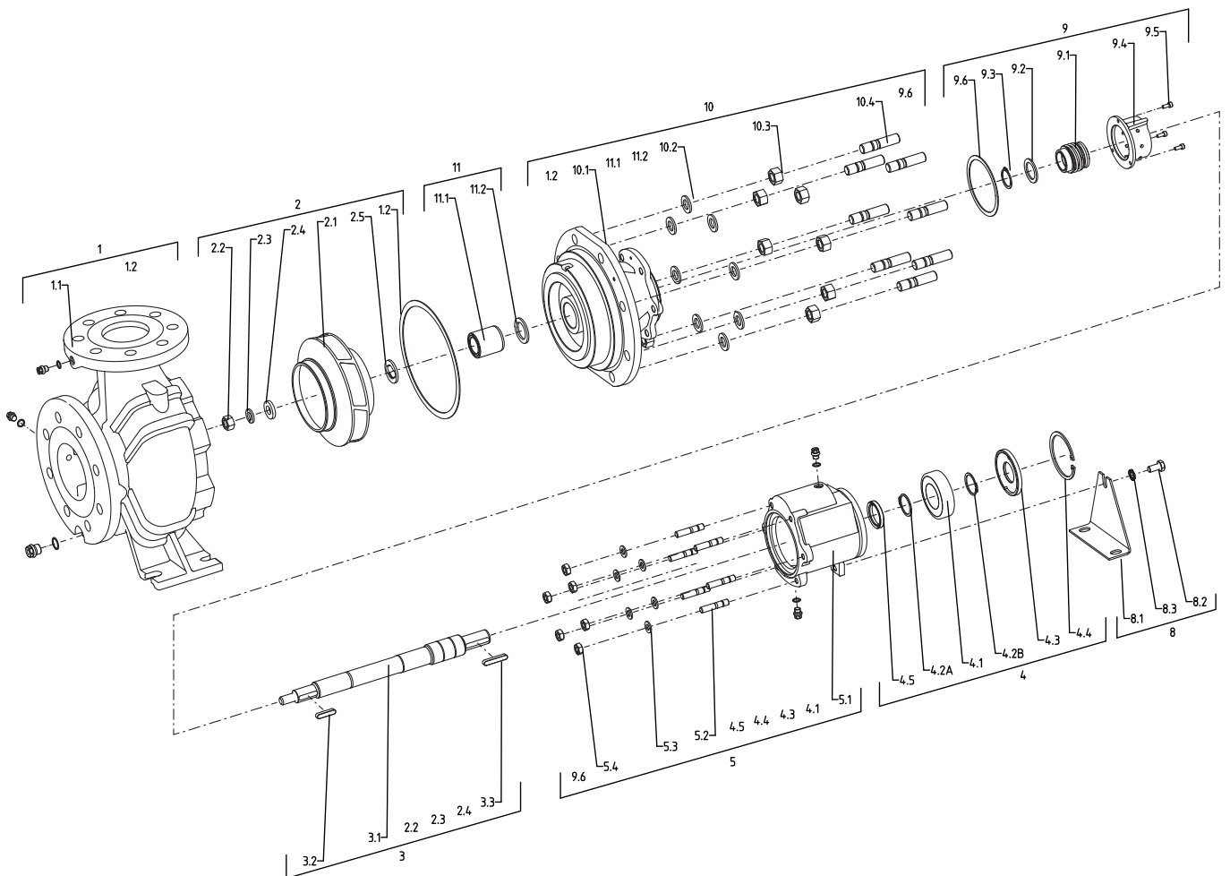
Fig. 32: Pumpe mit Gleitringdichtung
