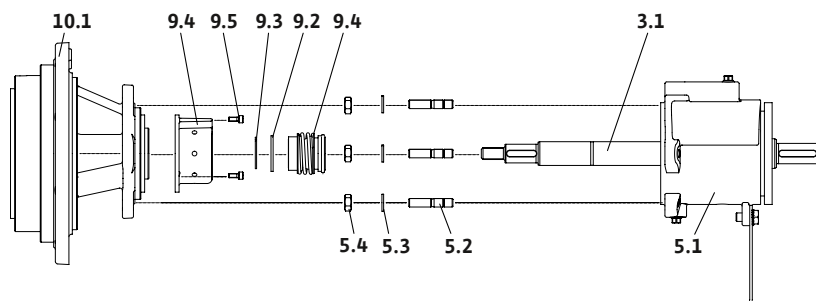
Fig. 22: Ausführung mit Gleitringdichtung
