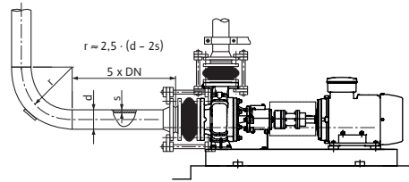
Fig. 10: Pumpe spannungsfrei anschließen, Beruhigungsstrecke vor und nach der Pumpe
