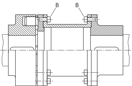
Fig. 18: Befestigungsschrauben B der Kupplungshälften
