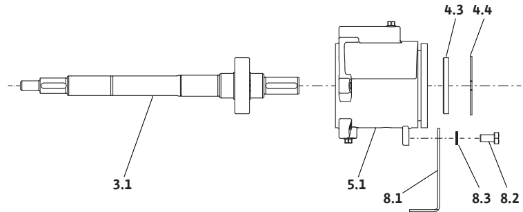
Fig. 26: Lagerträger
