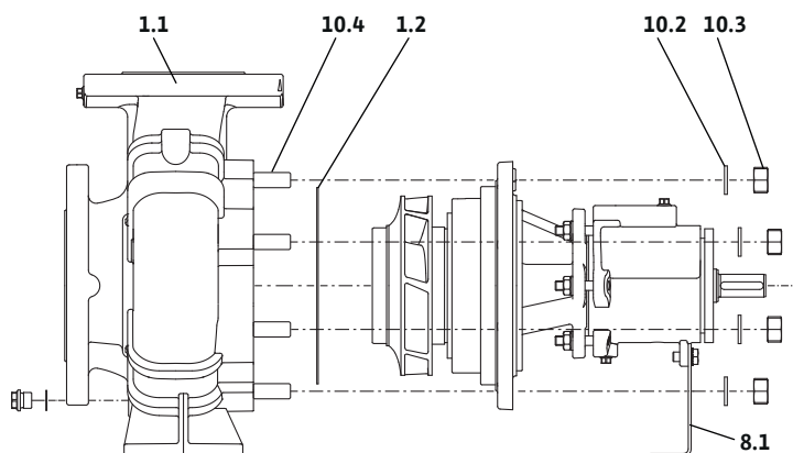
Fig. 30: Einschubeinheit einschieben
