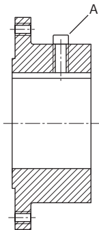
Fig. 17: Stellschraube A zur axialen Sicherung
