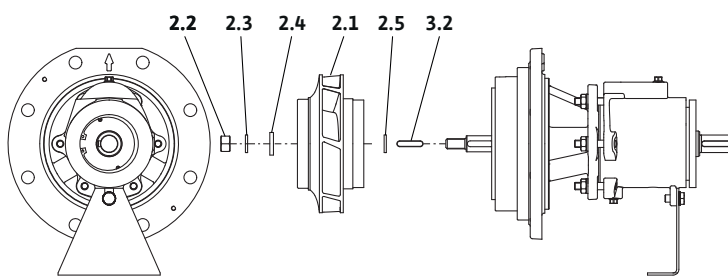
Fig. 29: Einschubeinheit montieren
