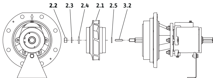
Fig. 20: Einschubeinheit demontieren
