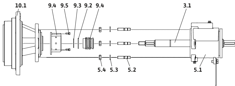
Fig. 27: Ausführung mit Gleitringdichtung
