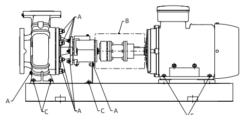
Fig. 31: Schraubenanzugsdrehmomente
