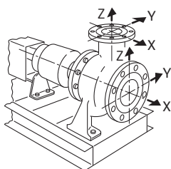
Fig. 3: Zulässige Kräfte und Momente an den Pumpenflanschen – Pumpe aus Grauguss EN-GJL-400-15, für Temperaturen bis 350 °C
