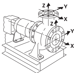
Fig. 8: Випадок навантаження 1A
