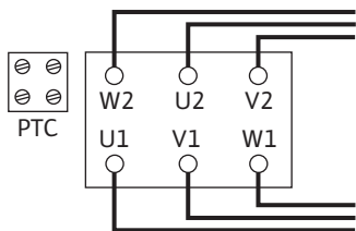
Fig. 16: Схема «зірка-трикутник»
