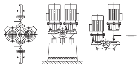
Fig. 4: Atmos GIGA-D nézet
