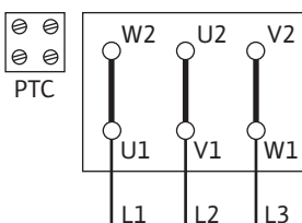
Fig. 14: Δ-kapcsolás
