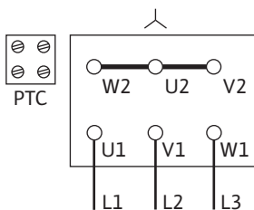
Fig. 15: Y-kapcsolás
