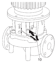
Fig. 17: A szerelő villa behelyezése
