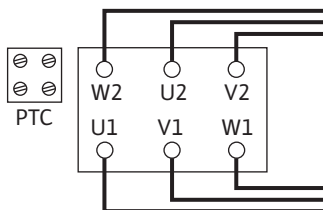
Fig. 16: Y-Δ-kapcsolás
