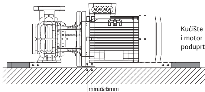
Fig. 42: Primeri montaže BL
