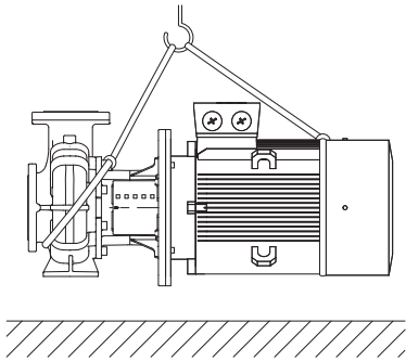
Fig. 33: Montaža omči za teret (verzija BL)
