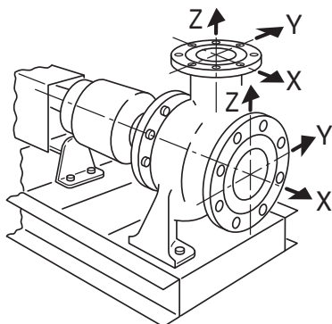
Fig. 39: Dozvoljene sile i momenti na priрубnicama pumpe – pumpa od sivog liva
