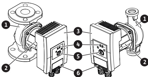
Fig. 1: Pumpun yleiskatsaus
